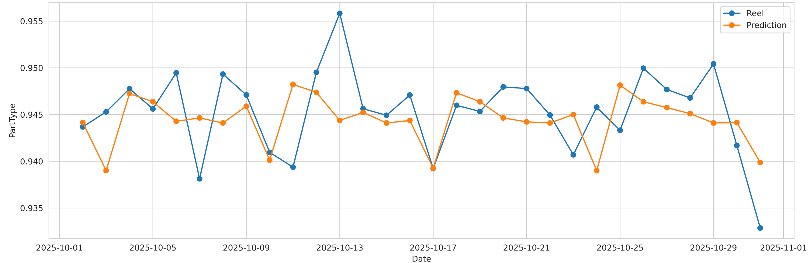
Exemple de prediction - Liaison 18124 - B
