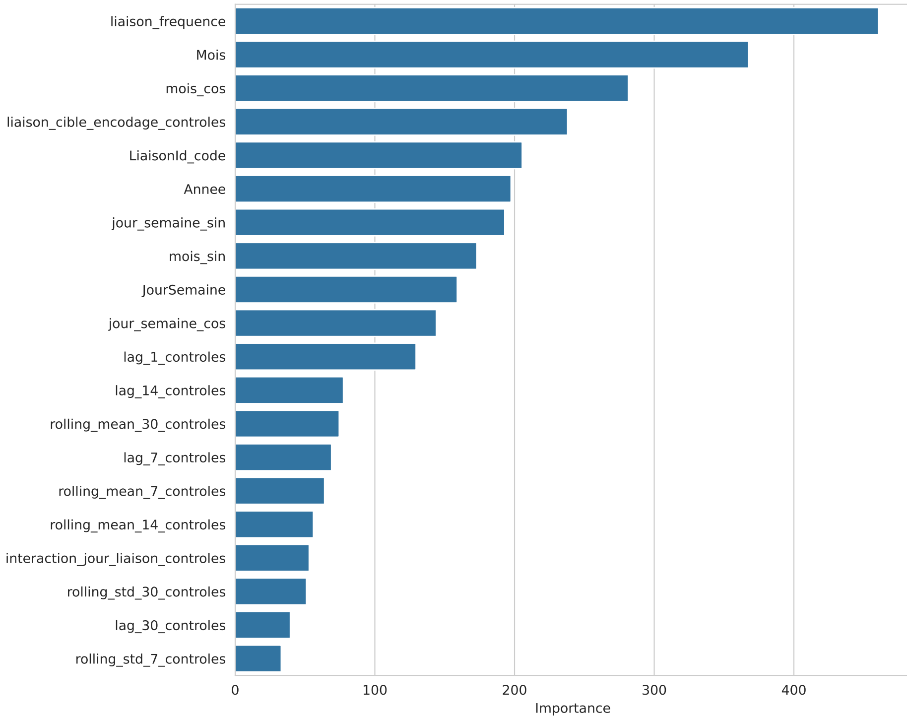
Importance moyenne des variables - LightGBM par categorie
