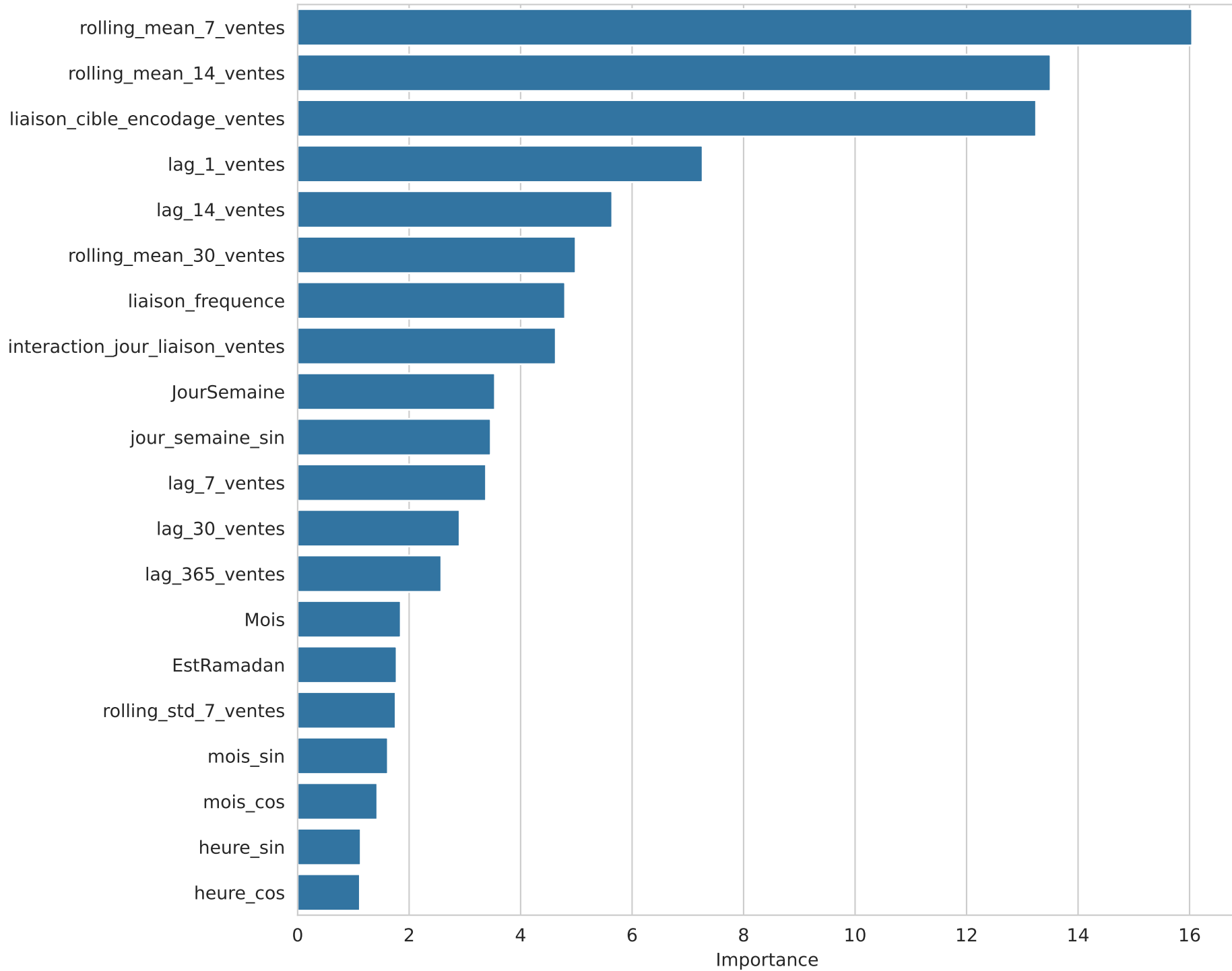
Importance des variables - CatBoost
