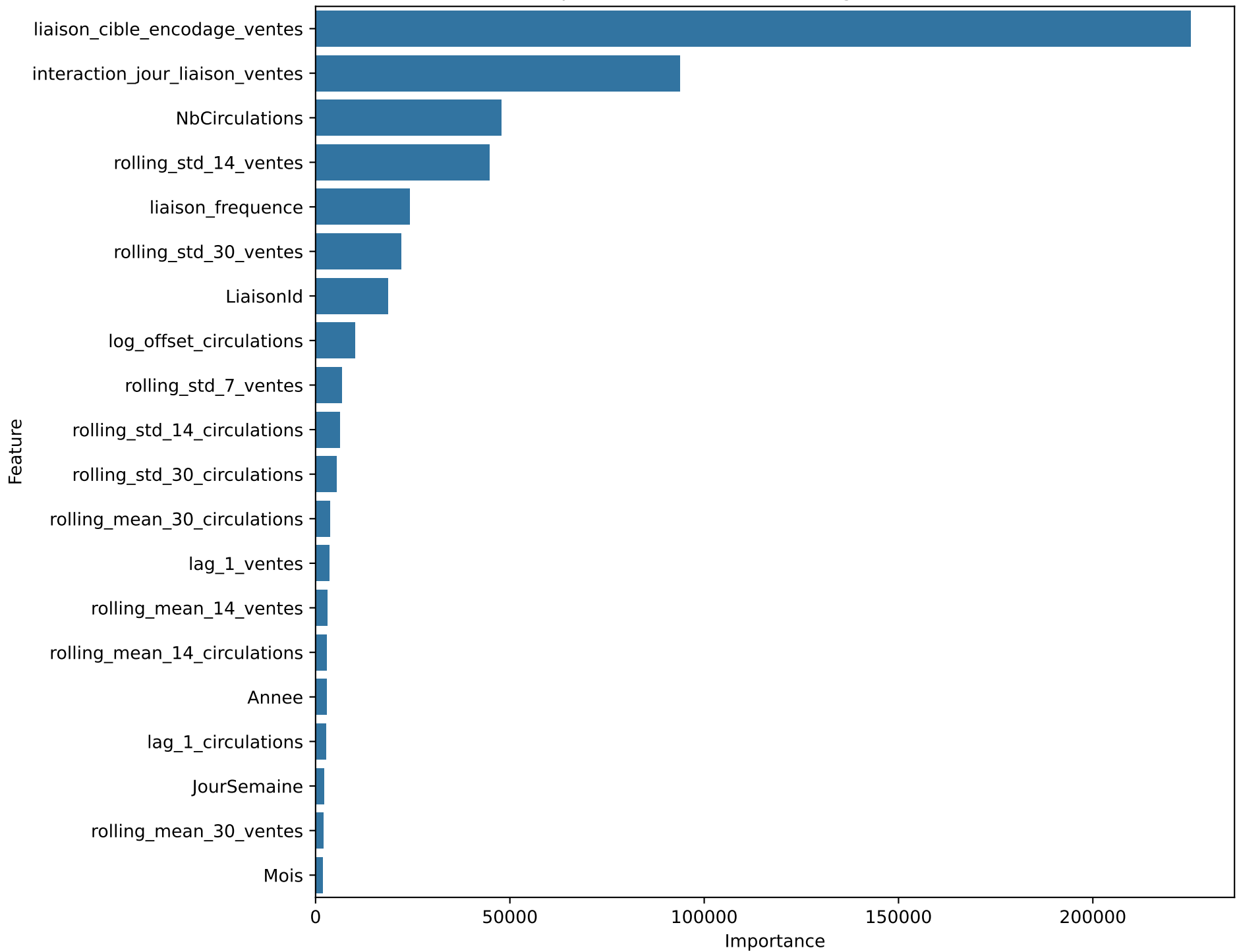
Importance des variables - LightGBM Tweedie
