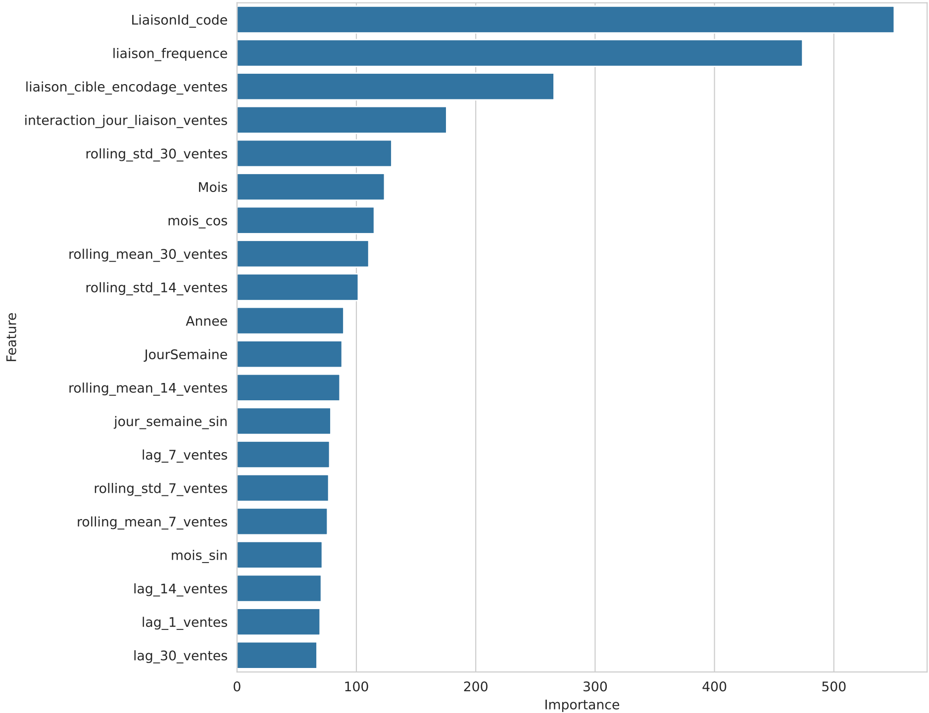
Importance moyenne des variables - LightGBM par categorie
