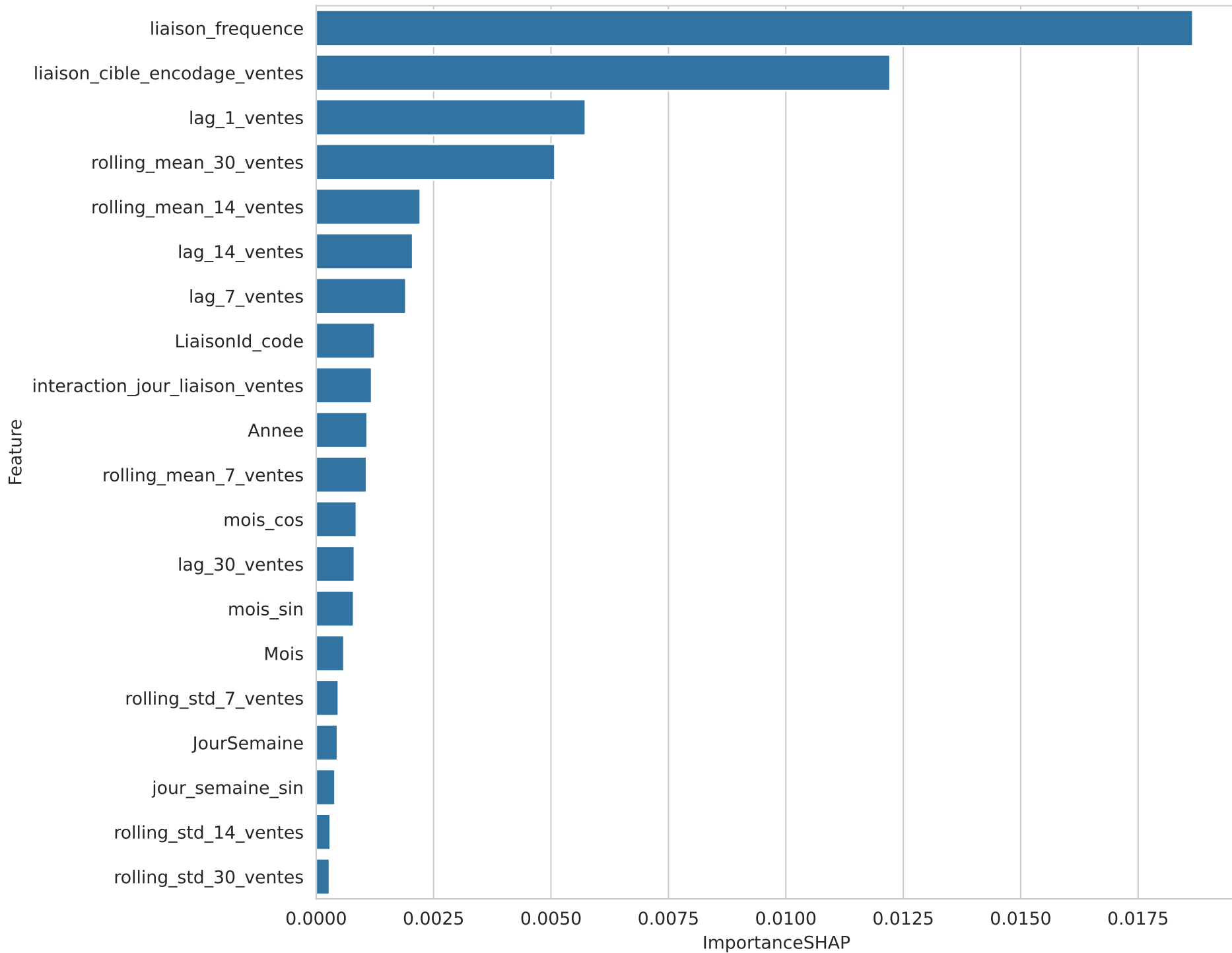
Importance SHAP moyenne - LightGBM par categorie
