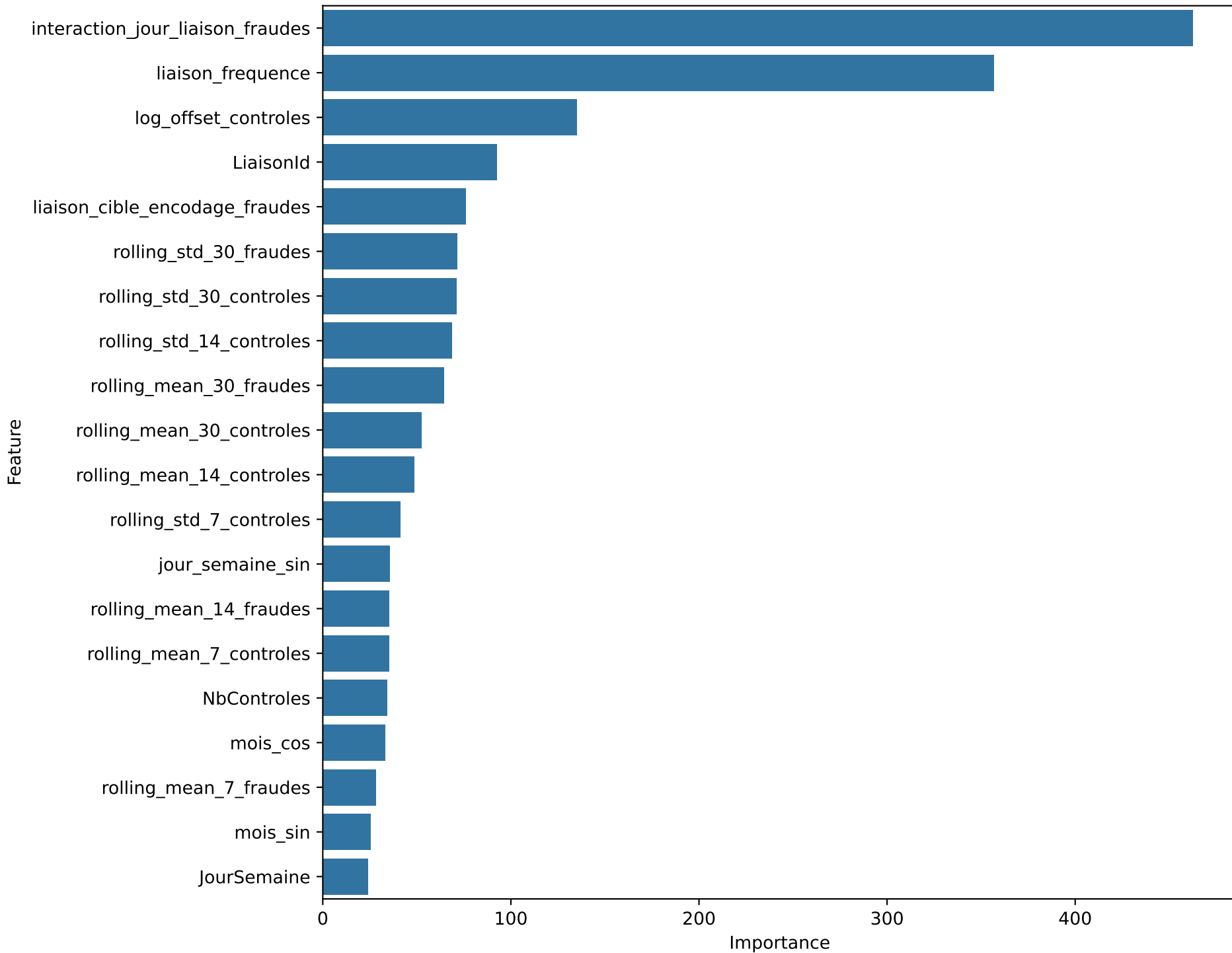
Importance des variables - LightGBM regression
