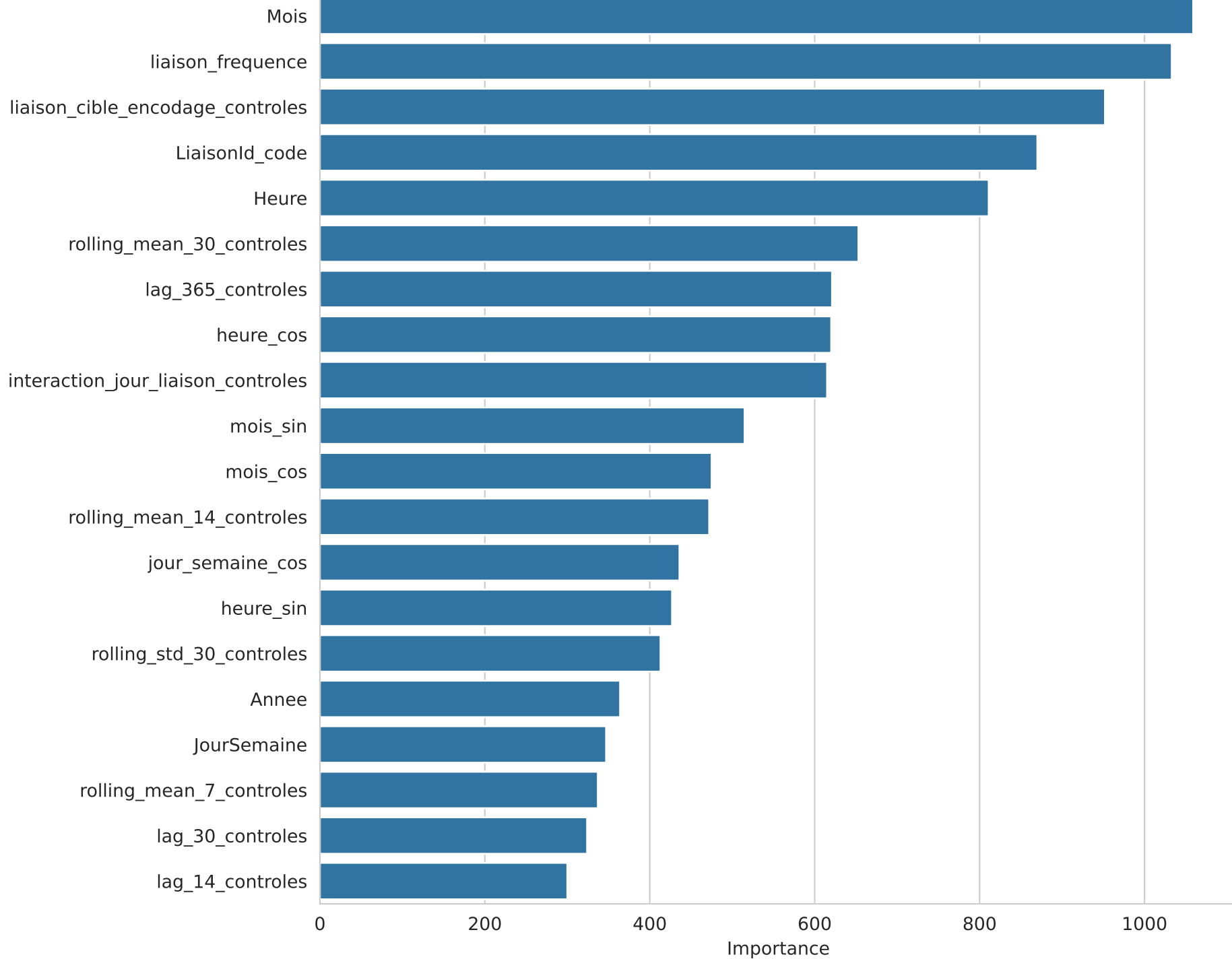
Importance des variables - LightGBM - J+30
