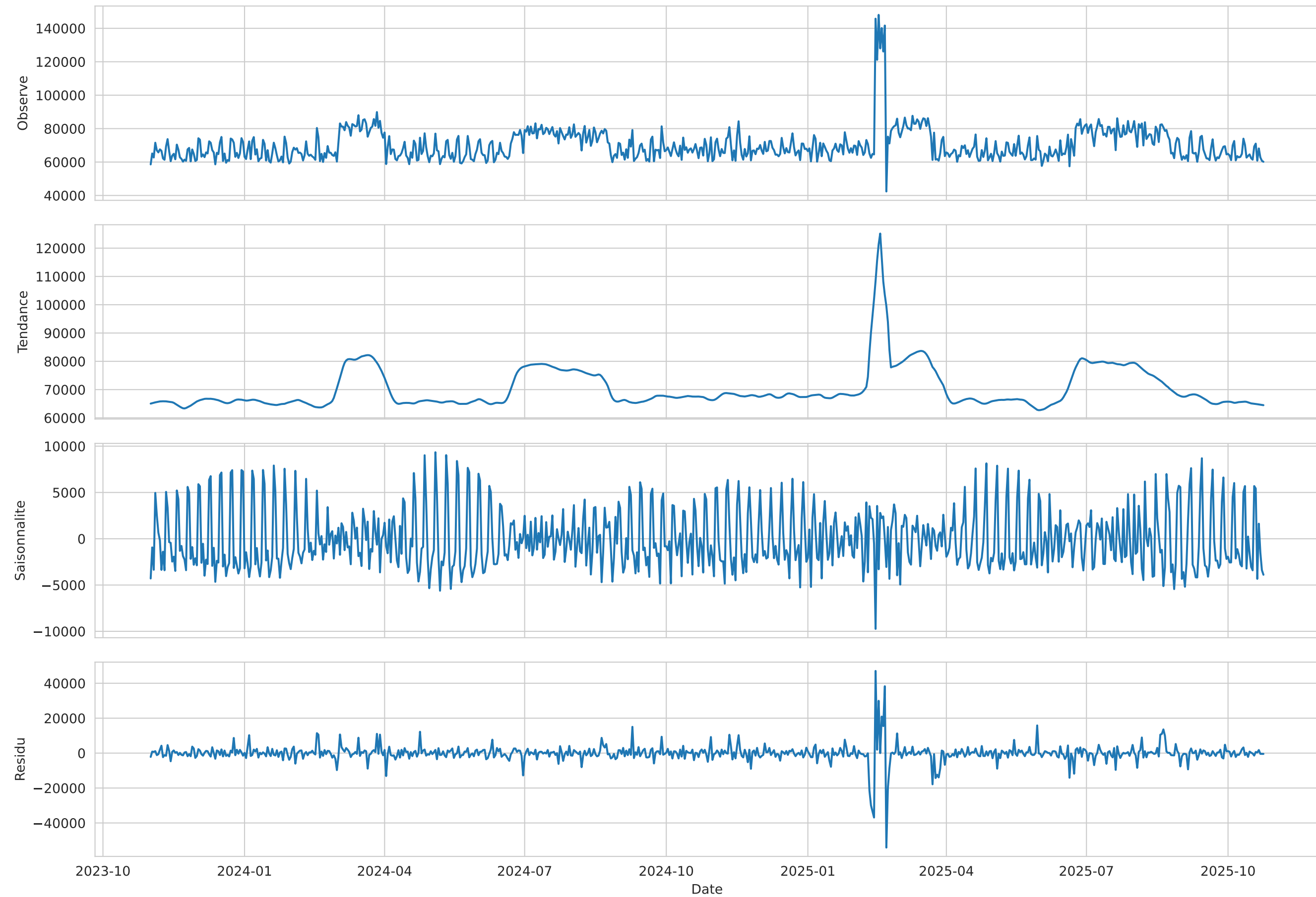
Decomposition STL - NbControles national quotidien - J+7
