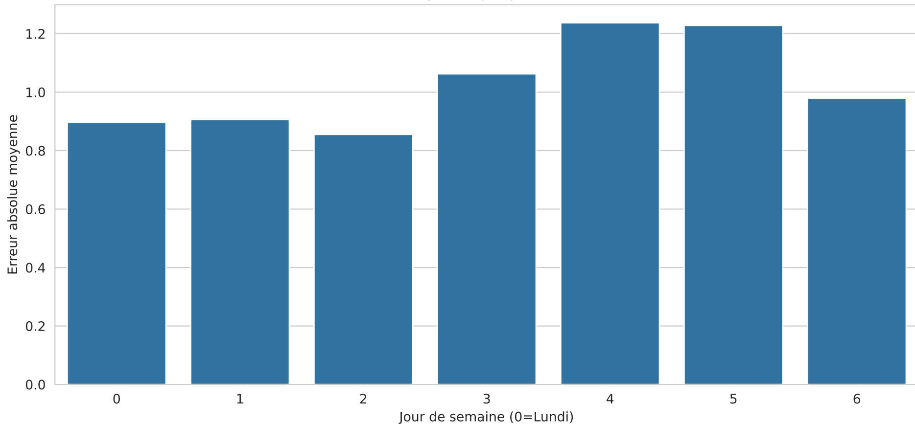
Erreur absolue moyenne par jour de semaine - J+15
