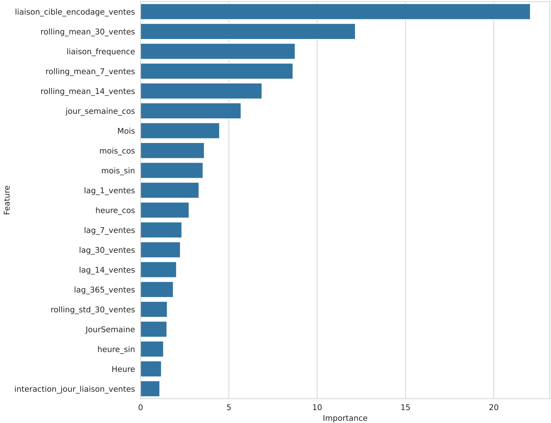
Importance des variables - CatBoost - J+30
