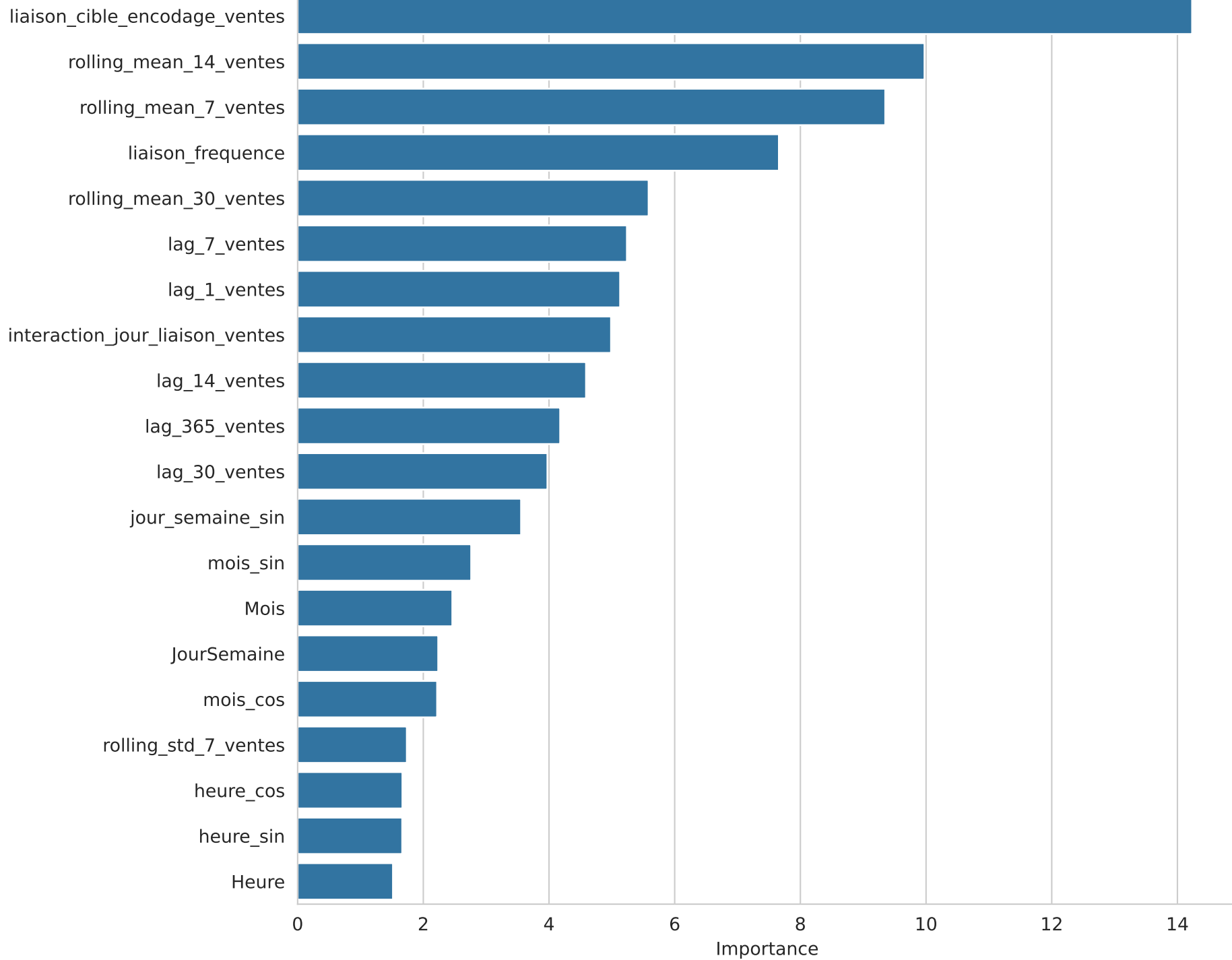
Importance des variables - CatBoost - J+7
