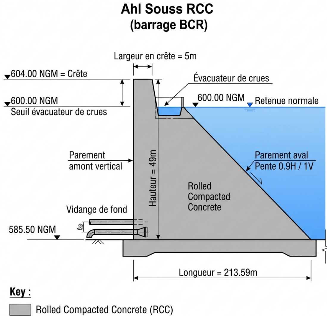
FIGURE 4-2 – Coupe transversale du barrage Ahl Souss (BCR) avec localisation de l'évacuateur de crues et de la vidange de fond.
