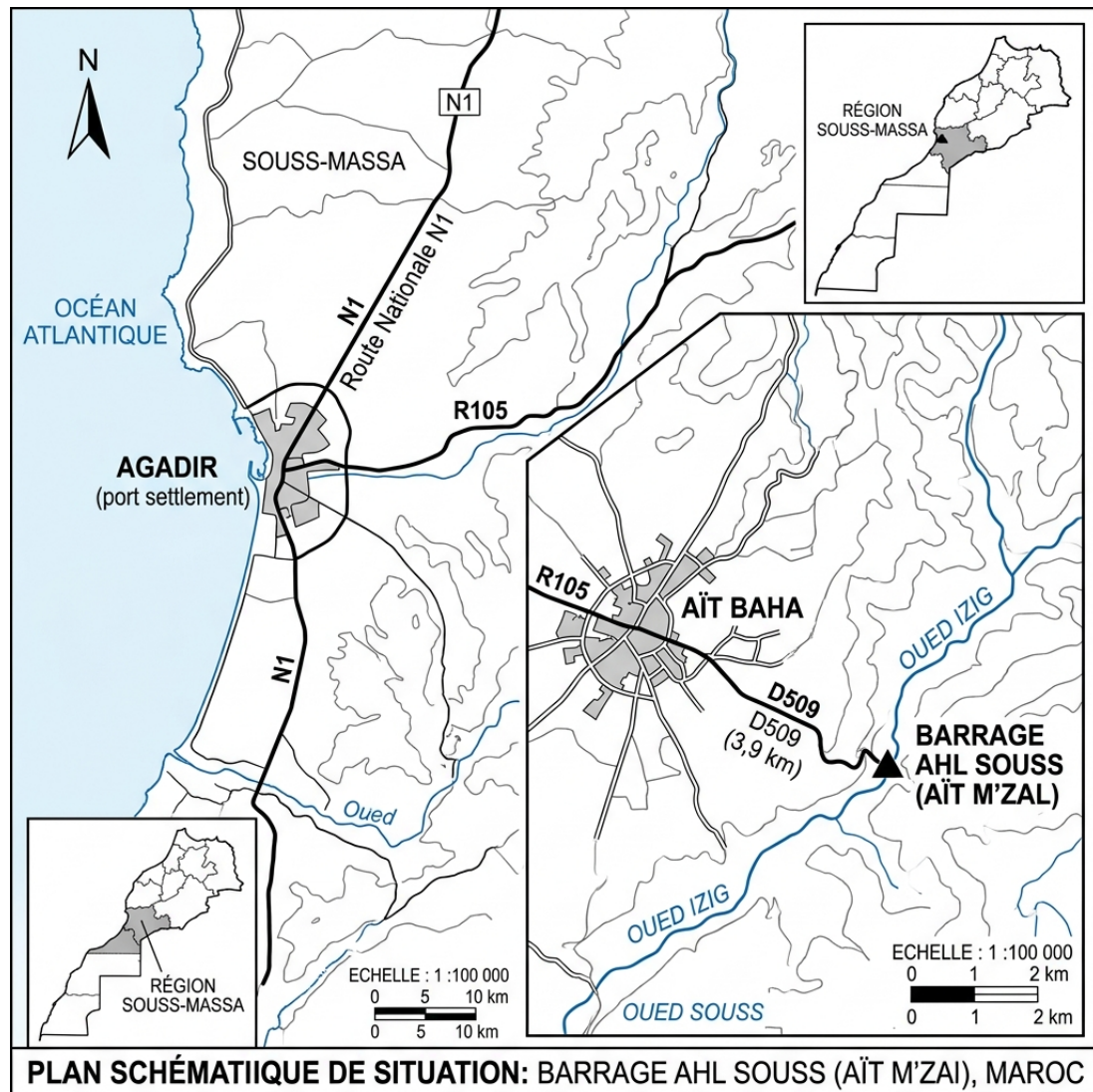
FIGURE 4-1 – Localisation du barrage Ahl Souss (Aït M'zal) sur l'oued Izig, province de Chtouka Aït Baha.
