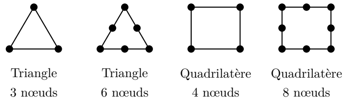
FIGURE 3-2 – Les géométries de référence de quelques éléments 2D courants.
