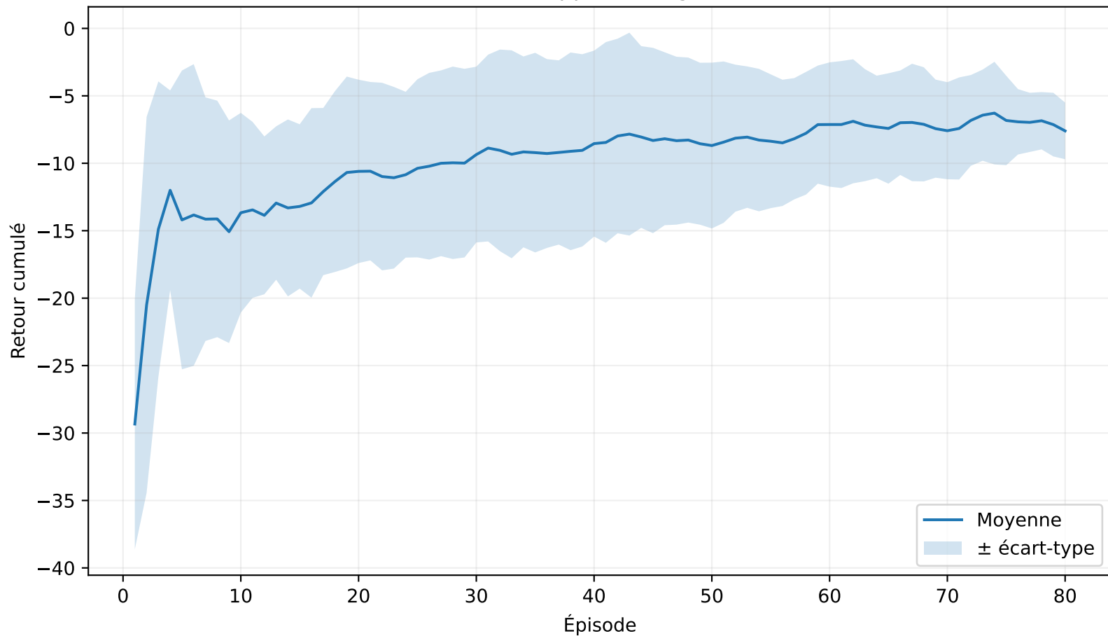
Courbe d'apprentissage DQN
