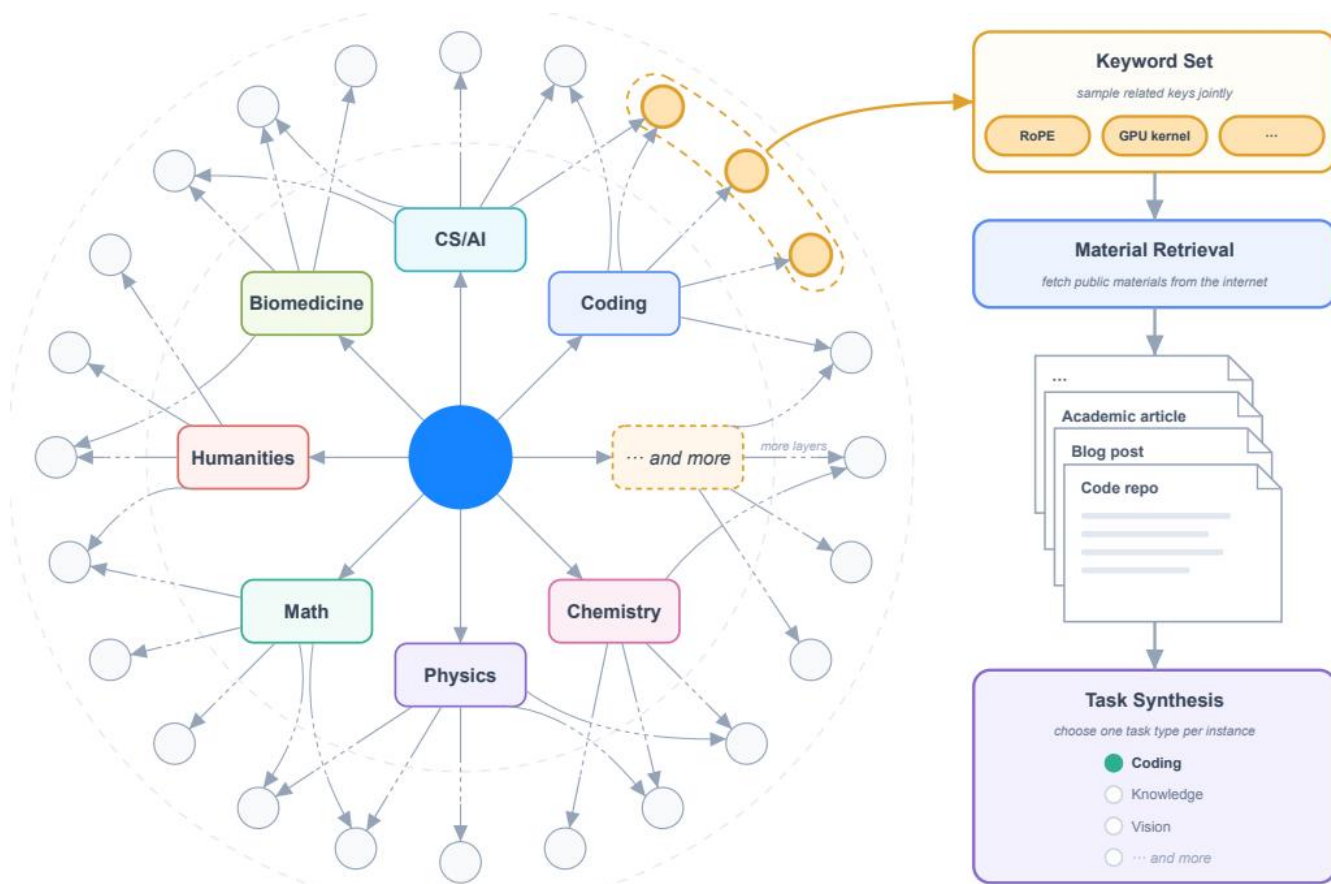
图 9: 知识图谱引导的任务合成概览。层次化组织的知识图谱在多个层级表示概念，范围从广泛领域到细粒度概念。相关节点被采样形成一个关键词集合，引导开源材料的检索。对于每个合成实例，系统选择一个任务类型，并使用检索到的材料合成相应的任务。
