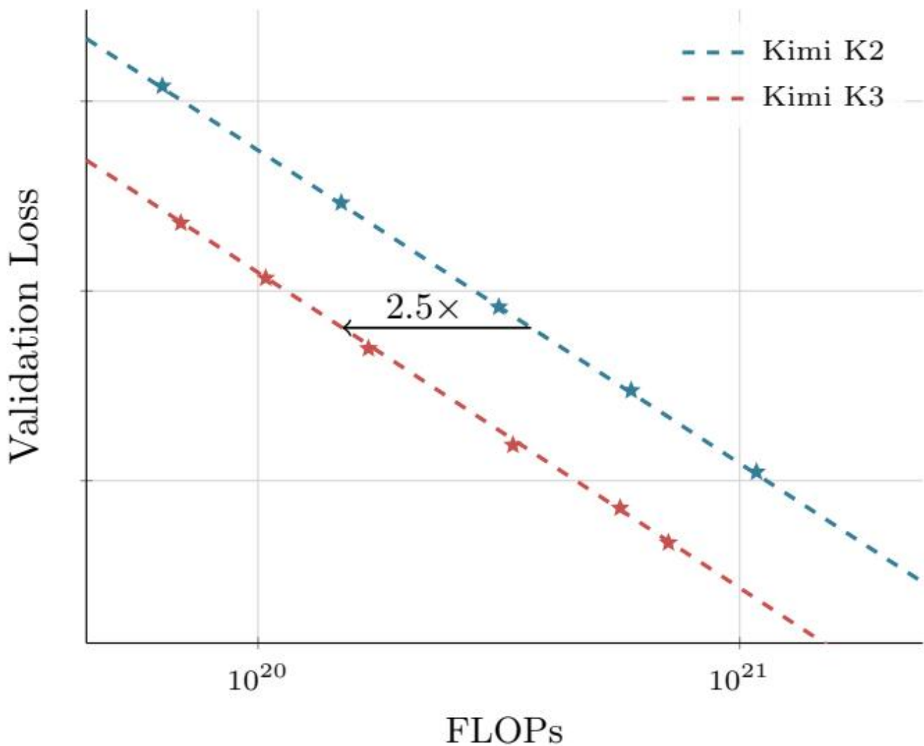
图 7: Kimi K2 和 Kimi K3 的拟合缩放定律曲线。Kimi K3 相比 Kimi K2 实现了 2.5 倍的缩放效率提升。
