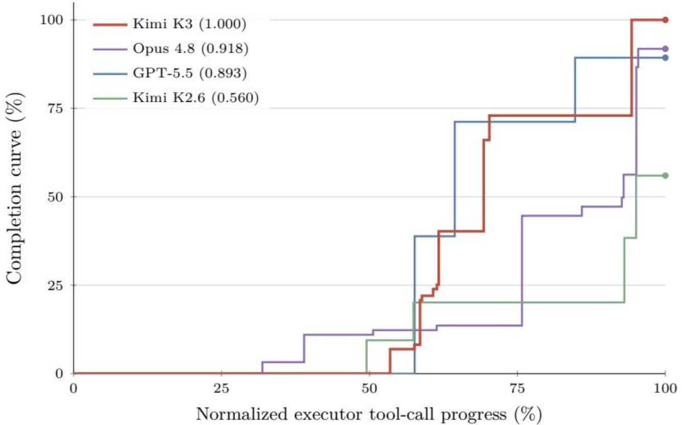
图 10: Camera Repair Management System 上的完成曲线，这是一个黑盒系统复现任务，智能体通过神谕 (oracle) 查询将一个隐藏的 3D 相机维修系统重建为 Web 应用。完成度表示验证器评估的任务进度。
