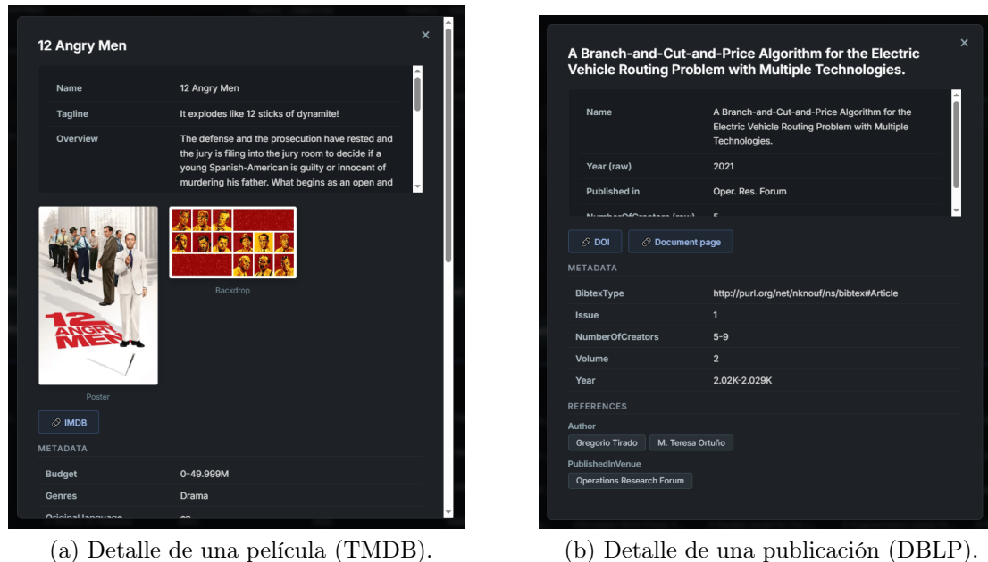
Figura 5.4: Modal de detalle de una entidad sobre cada dominio.
