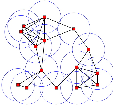
Figure – Exemple de graphe unitaire
