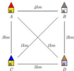
(a) Instance du problème
