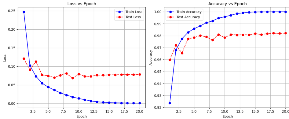
Figure 8: Courbe de perte (Loss) et de précision (Accuracy) sur les données d'entraînement (60 000 images) et validation (10 000 images).
