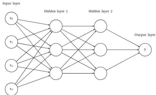
Figure – Structure hiérarchique du MLP
