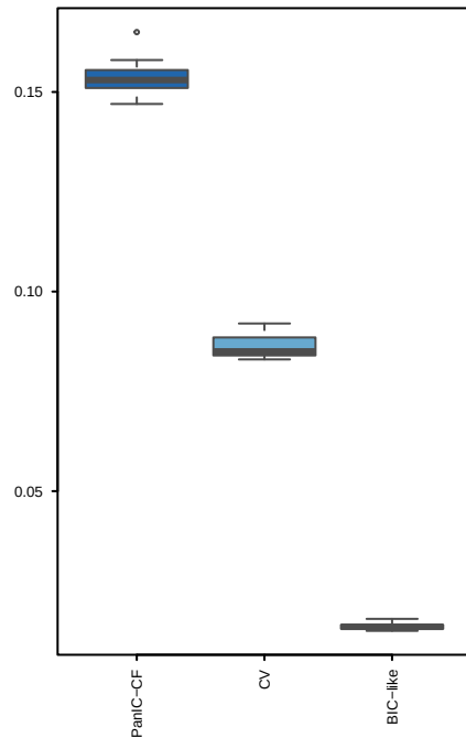
Poisson
