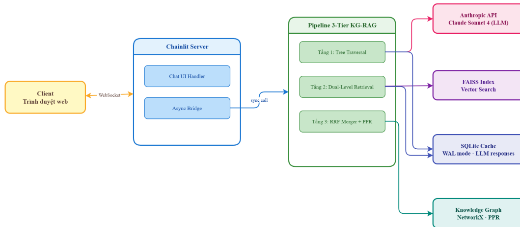
Hình 4.1: Kiến trúc triển khai hệ thống: Client (trình duyệt web) kết nối với máy chủ Chainlit qua WebSocket, máy chủ gọi pipeline 3-Tier KG-RAG đồng bộ thông qua Async Bridge, pipeline truy vấn các dịch vụ ngoại vi gồm Anthropic API (LLM), FAISS Index (vector search) và SQLite Cache (LLM response caching).
