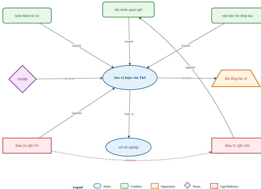
Hình 3.2: Đồ thị con minh họa các thực thể và quan hệ xung quanh chủ đề “bảo vệ luận văn thạc sĩ”. Các nút được phân loại theo ontology (Action, Condition, Organization, Person, Legal Reference) và các cạnh thể hiện các loại quan hệ (requires, leads_to, regulates, references).
