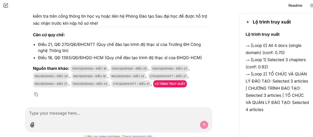
Hình 4.6: Lộ trình truy xuất 3 vòng lặp: Loop 0 chọn tài liệu, Loop 1 chọn chương, Loop 2 truy xuất điều khoản
