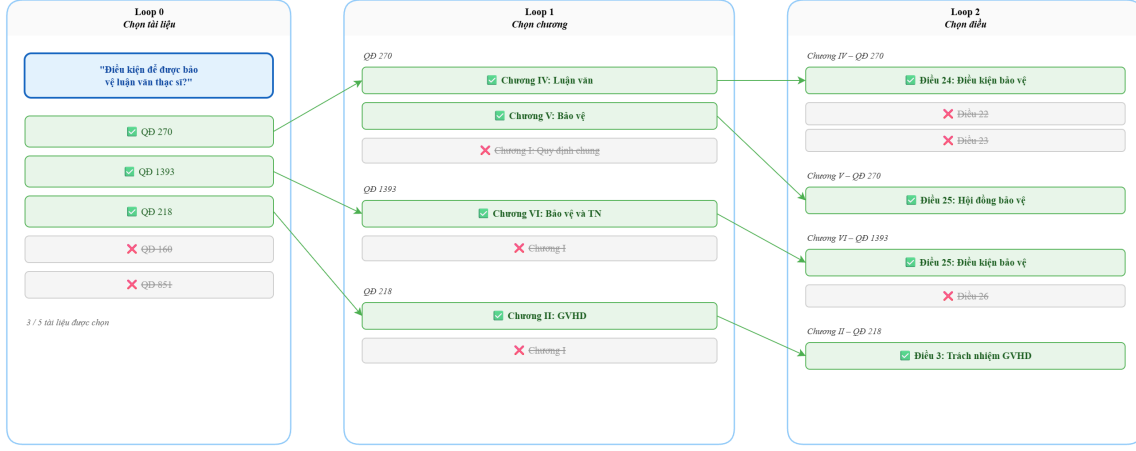
Hình 3.6: Minh họa quá trình duyệt cây ba vòng lặp với truy vấn “Điều kiện để được bảo vệ luận văn thạc sĩ?”. Các nút xanh là được chọn bởi LLM, các nút xám bị loại. Loop 0 chọn 3/5 tài liệu, Loop 1 thu hẹp xuống các chương liên quan, Loop 2 xác định các điều khoản cụ thể.
