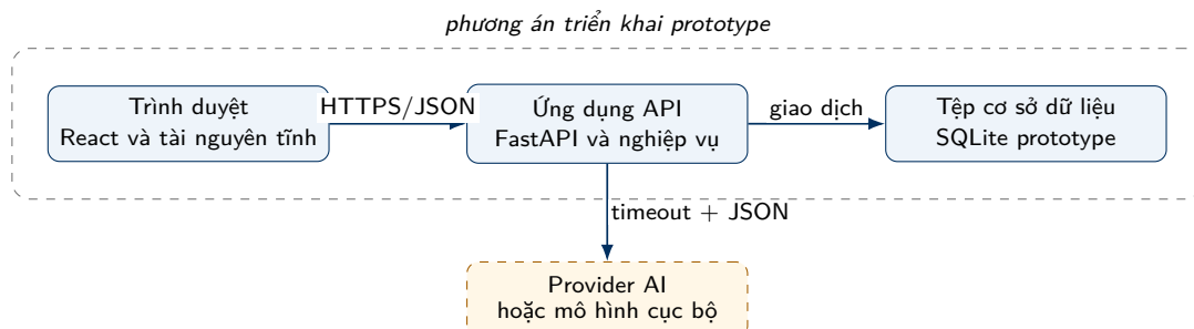
Hình 7.1: Phương án triển khai prototype
