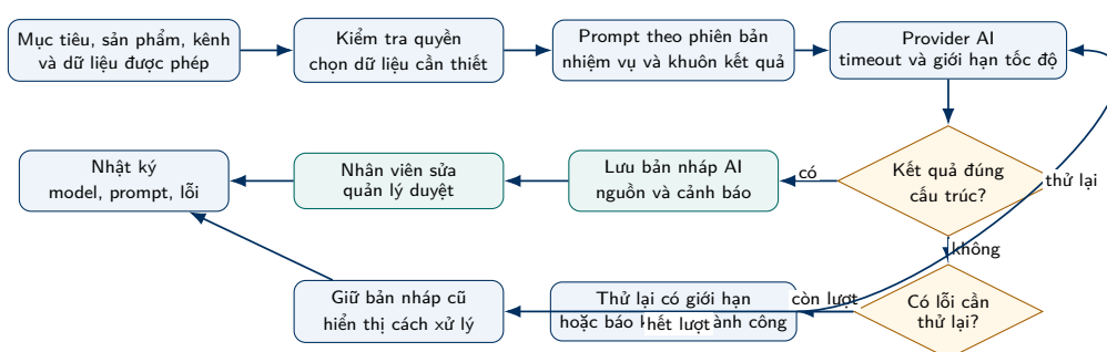
Hình 6.1: Luồng xử lý một yêu cầu AI
