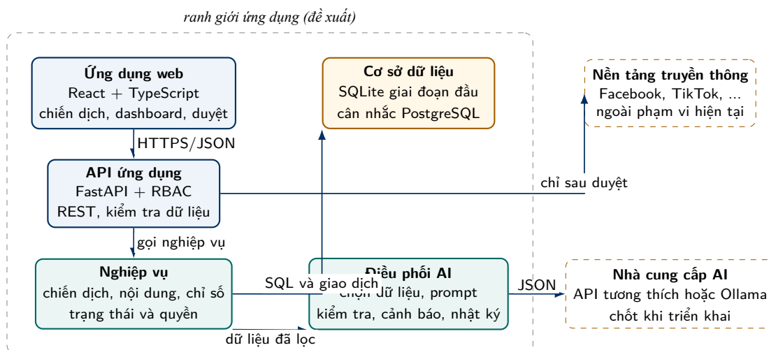
Hình 4.1: Sơ đồ khối logic và dòng dữ liệu của hệ thống
