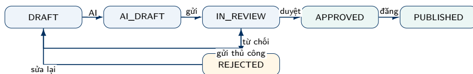
Hình 5.3: Vòng đời dự kiến của một bản nội dung
