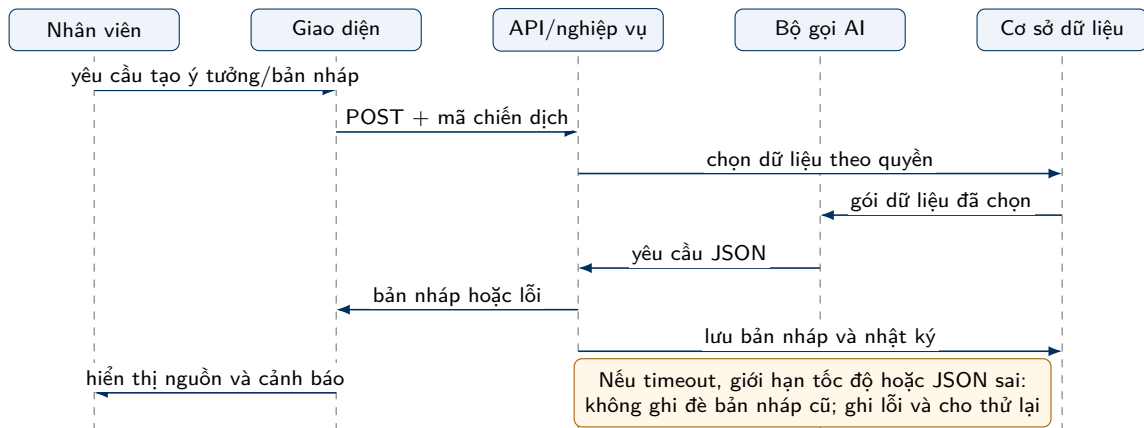
Hình 5.4: Trình tự tạo bản nháp AI
