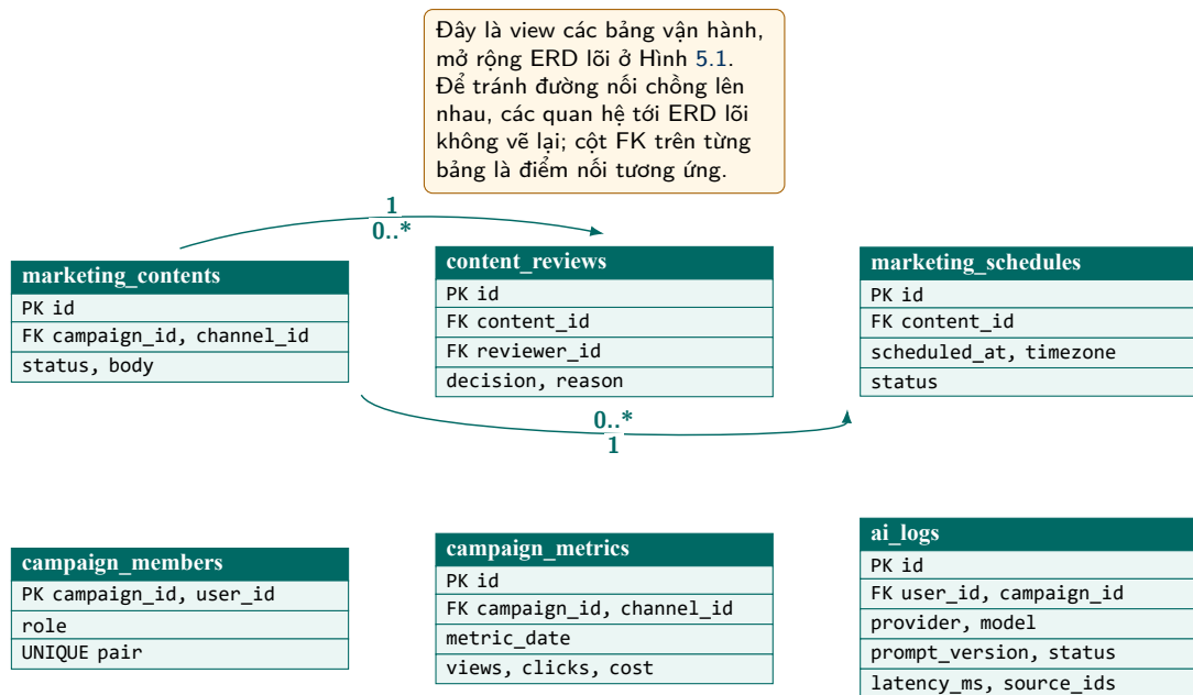
Hình 5.2: Các bảng vận hành và điểm nối tới ERD lỗi
