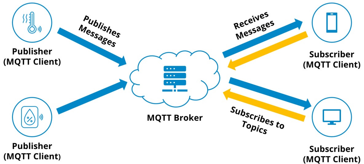
Hình 3.8: Giao thức MQTT trong hệ thống nhúng
