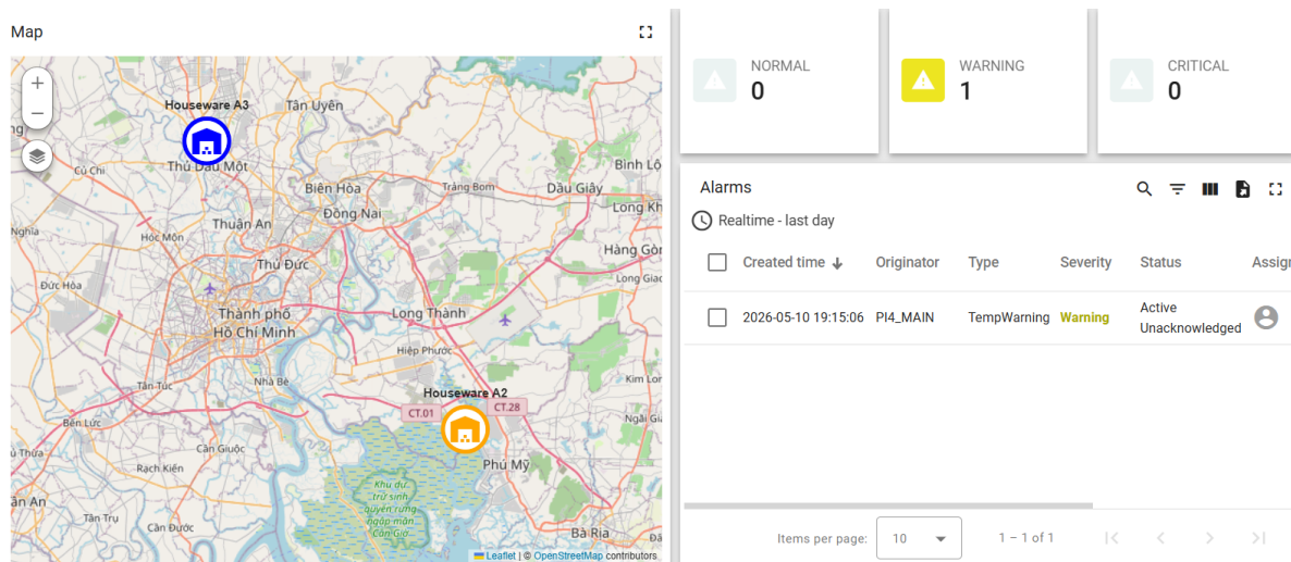
Hình 4.1: Trang chủ Dashboard CoreIoT
