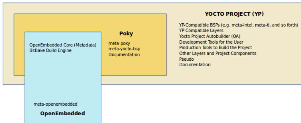
Hình 2.3: Tổng thể hệ sinh thái Yocto Project
