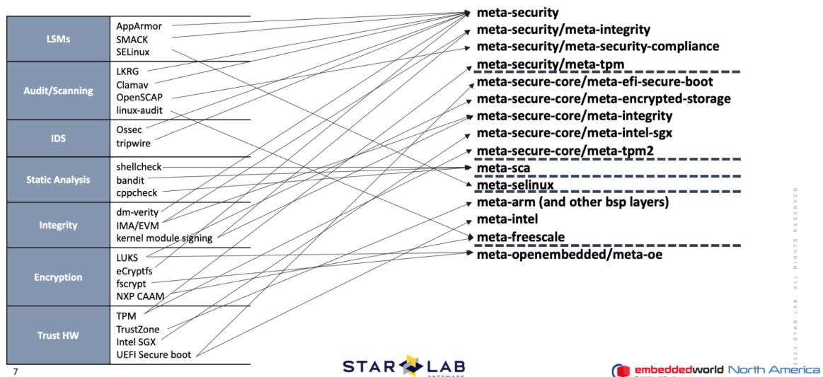
Hình 3.1: Tăng cường bảo mật cho hệ thống nhúng Yocto là một bài toán đa khía cạnh Nguồn: Star Lab Software
