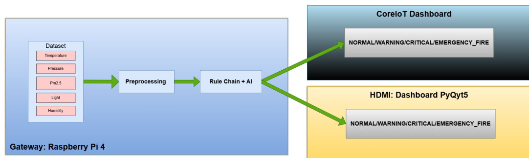
Hình 4.2: Kiến trúc khối xử lý cảnh báo trên gateway Raspberry Pi 4
