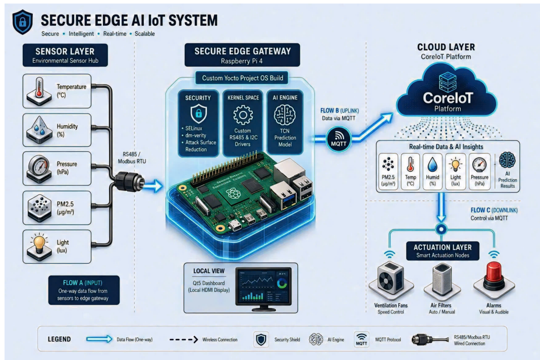
Hình 1.3: Kiến trúc tổng thể của hệ thống
