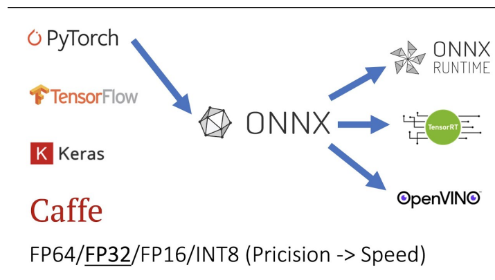
Hình 3.9: Định dạng ONNX
