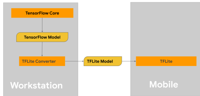
Hình 3.10: Định dạng TensorFlow Lite
