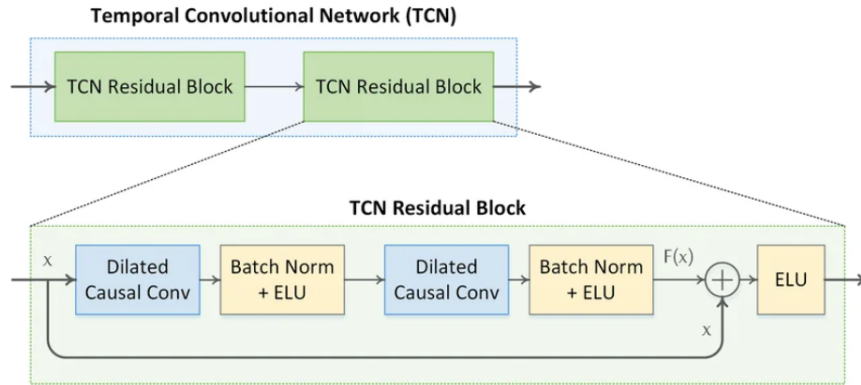
Hình 4.3: mô hình TCN
