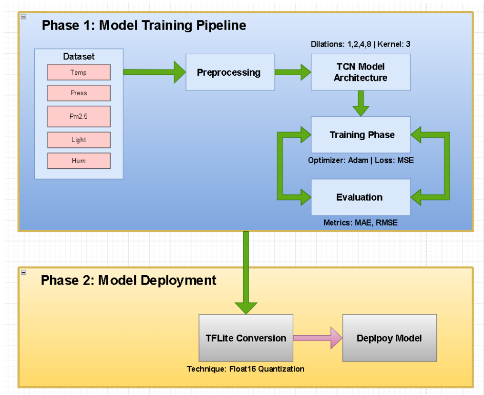
Hình 4.2: Sơ đồ khối Module AI
