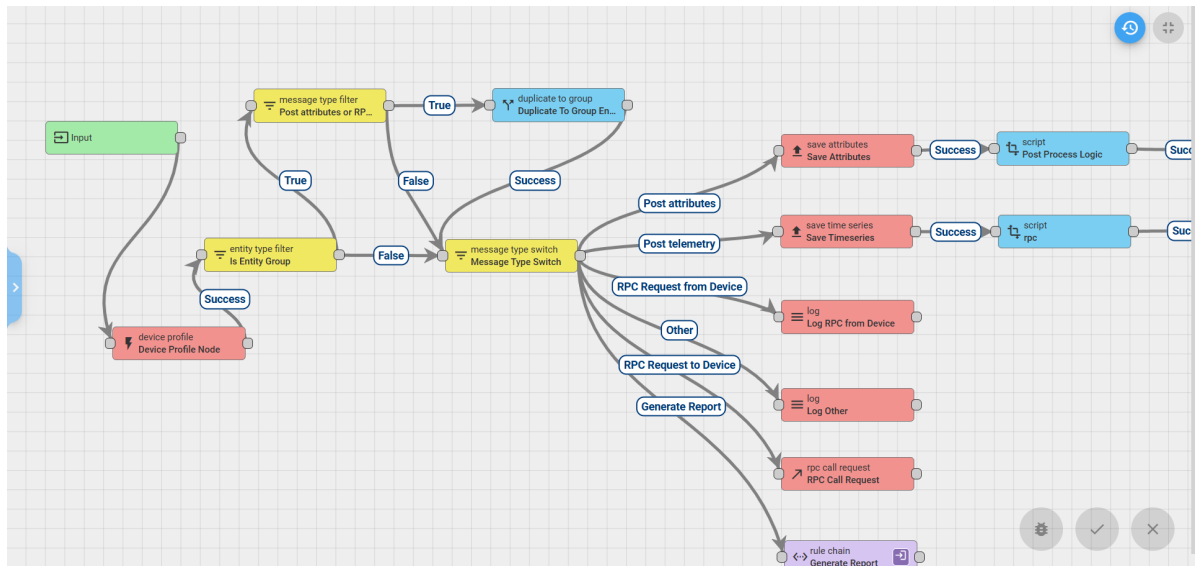
Hình 3.14: Xây dựng quy tắc xử lý dữ liệu và sự kiện trong CoreIoT
