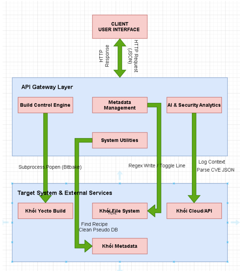
Hình 4.5: Sơ đồ khối Tool
