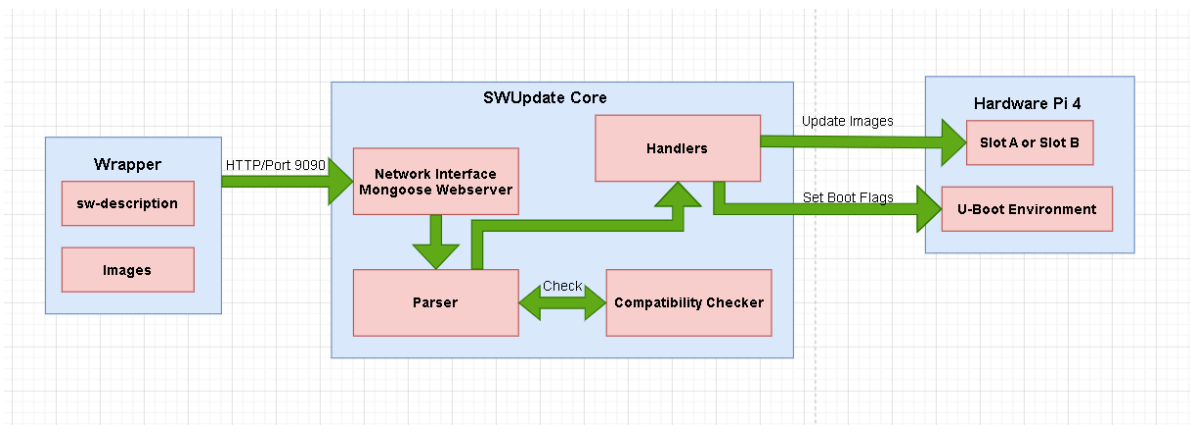
Hình 4.4: Sơ đồ khối OTA
