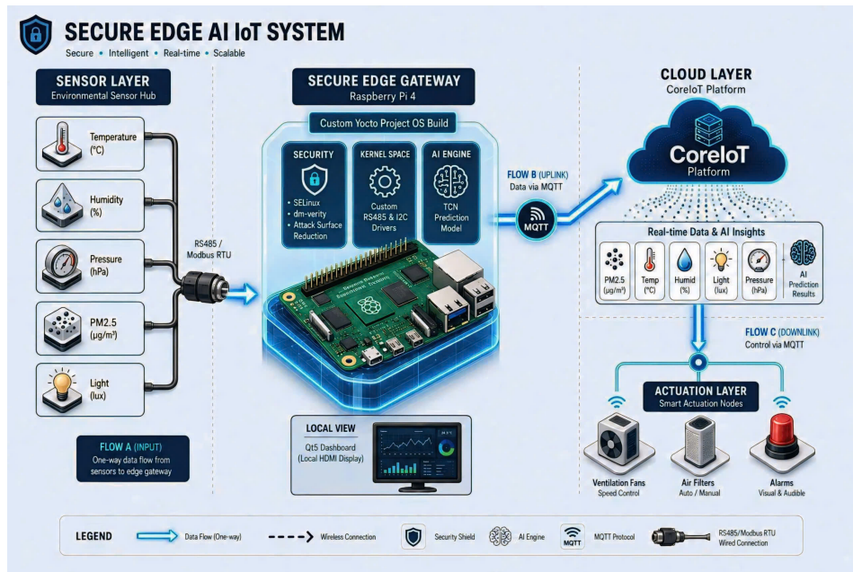
Hình 4.1: Sơ đồ kiến trúc hệ thống
