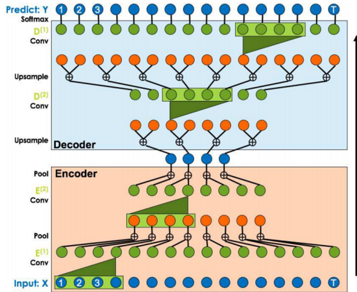
Hình 3.8: Kiến trúc mô hình TCN
