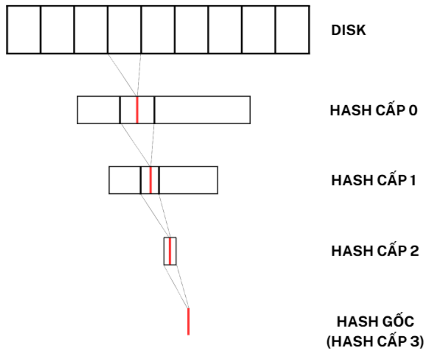
Hình 3.6: Bảo mật chống tấn công offline với dm-verity trong Yocto
