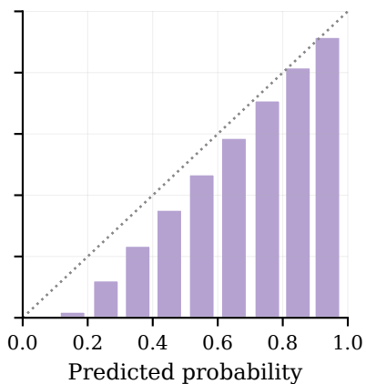
Vistral SFT ECE=0.072
