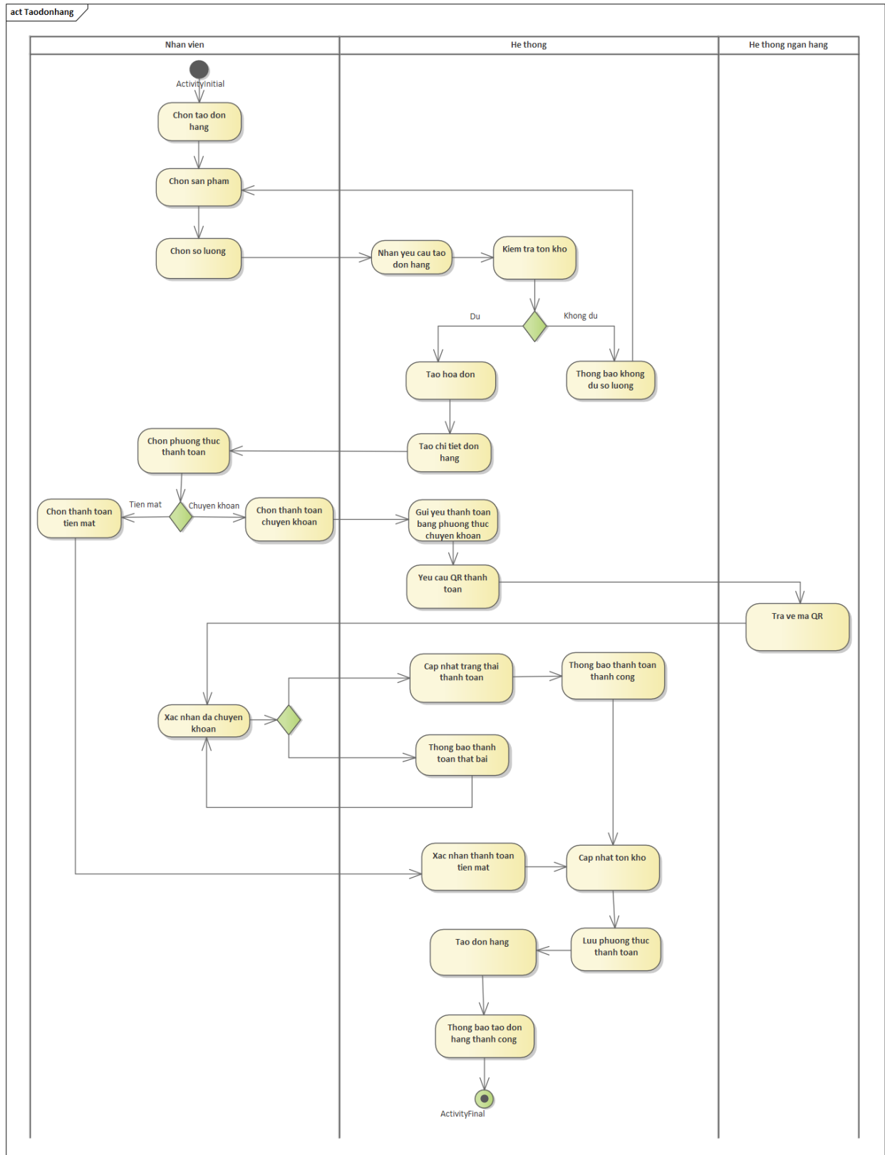
Hình 3. 4 Sơ đồ hoạt động Tạo đơn hàng
