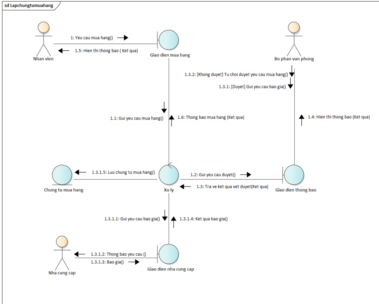
Hình 3. 17 Sơ đồ cộng tác Lập chứng từ mua hàng
