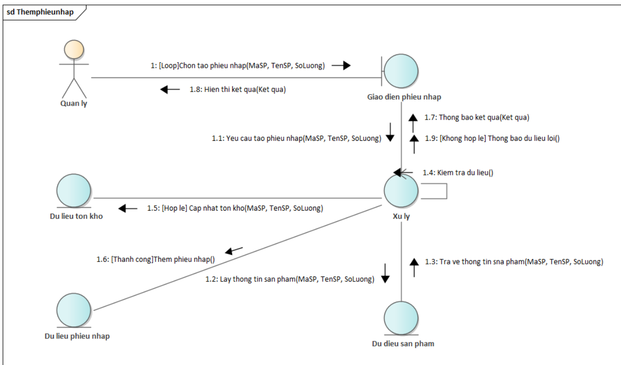
Hình 3. 19 Sơ đồ cộng tác Thêm phiếu nhập
