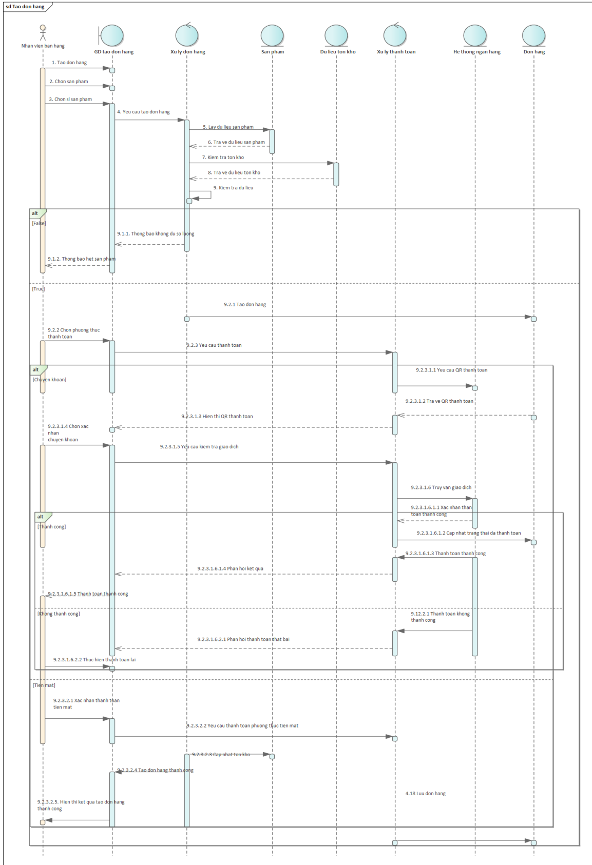
Hình 3. 10 Sơ đồ tuần tự tạo đơn hàng
