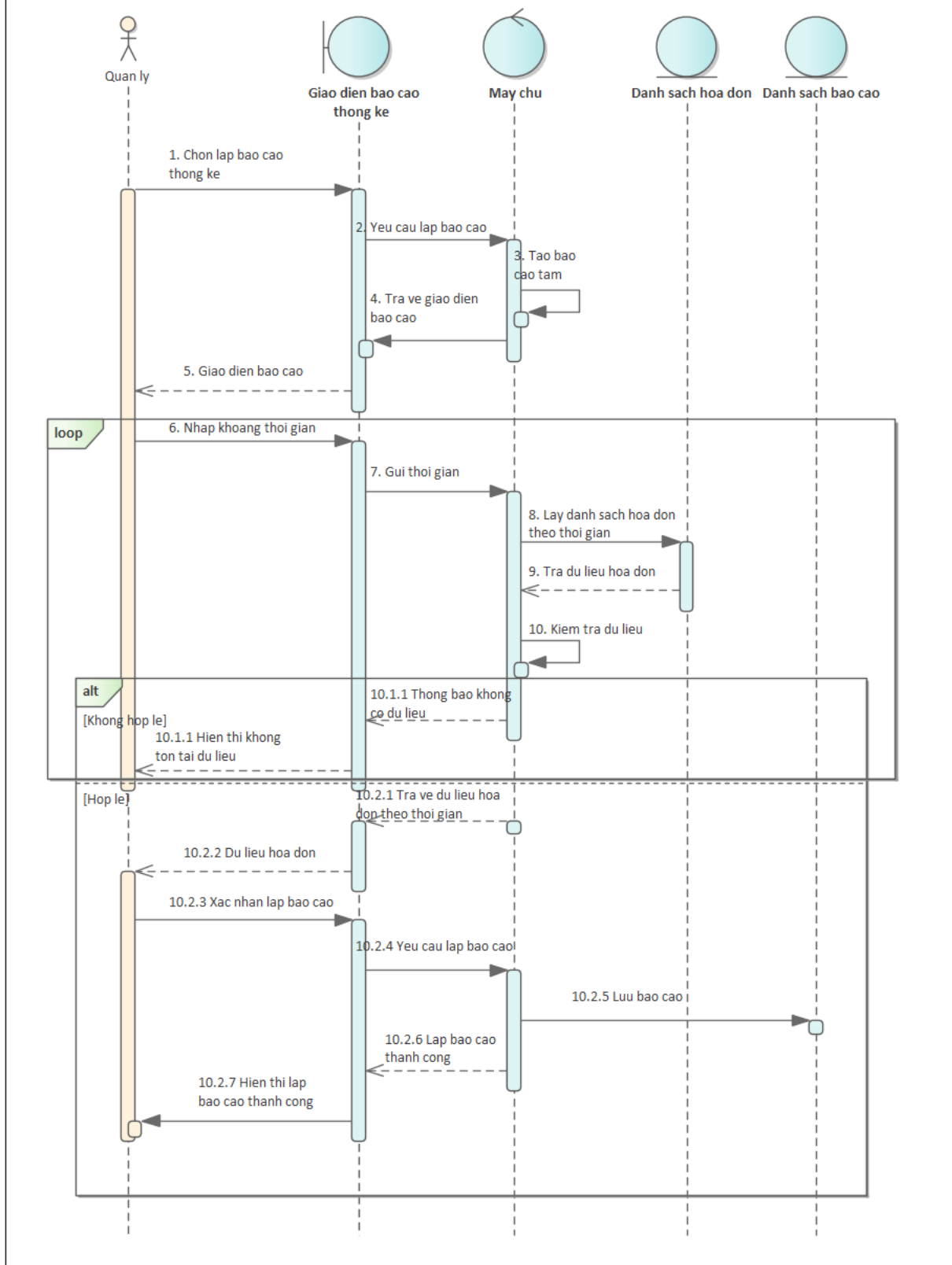
Hình 3. 12 Sơ đồ tuần tự Lập báo cáo thống kê
