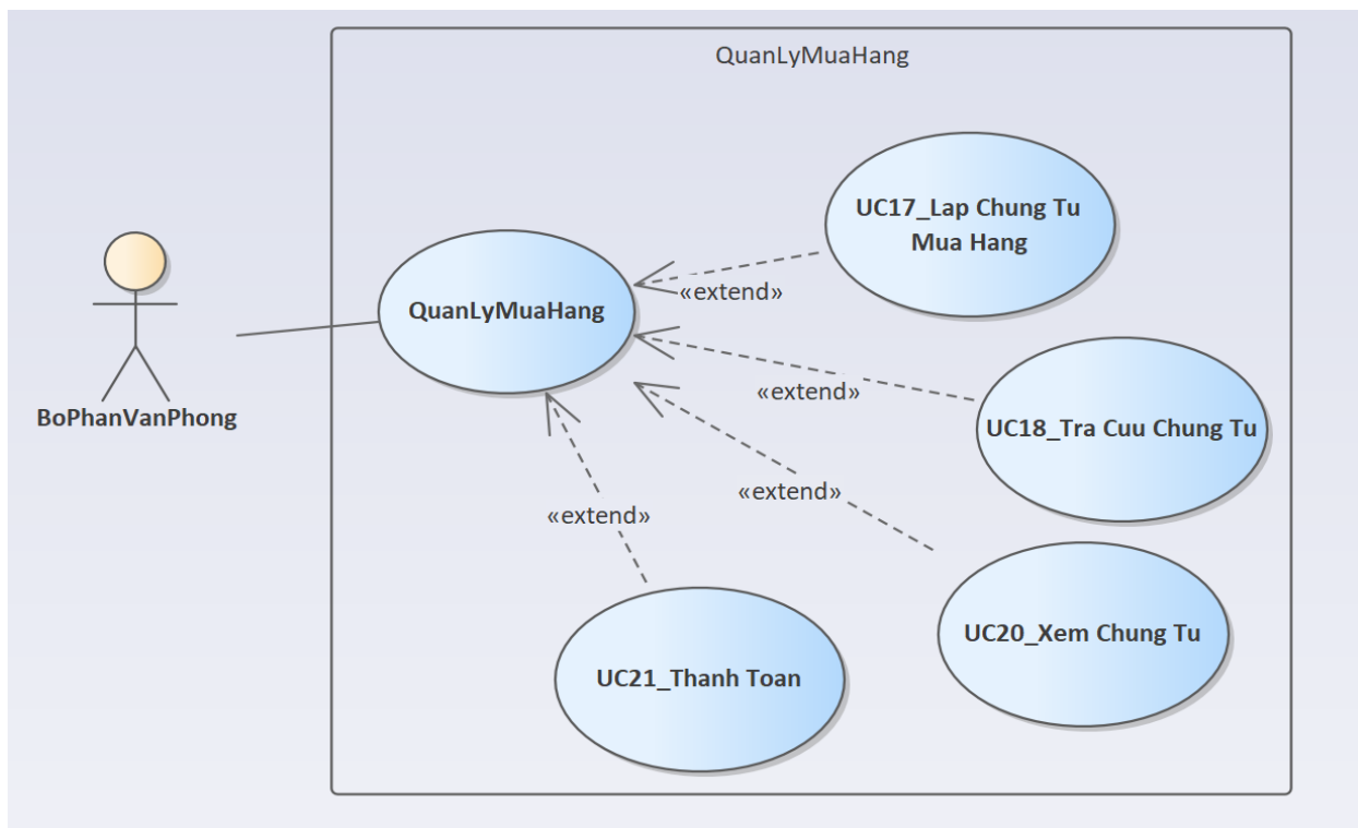
Hình 2. 6. Sơ đồ Use Case Quản lý mua hàng
