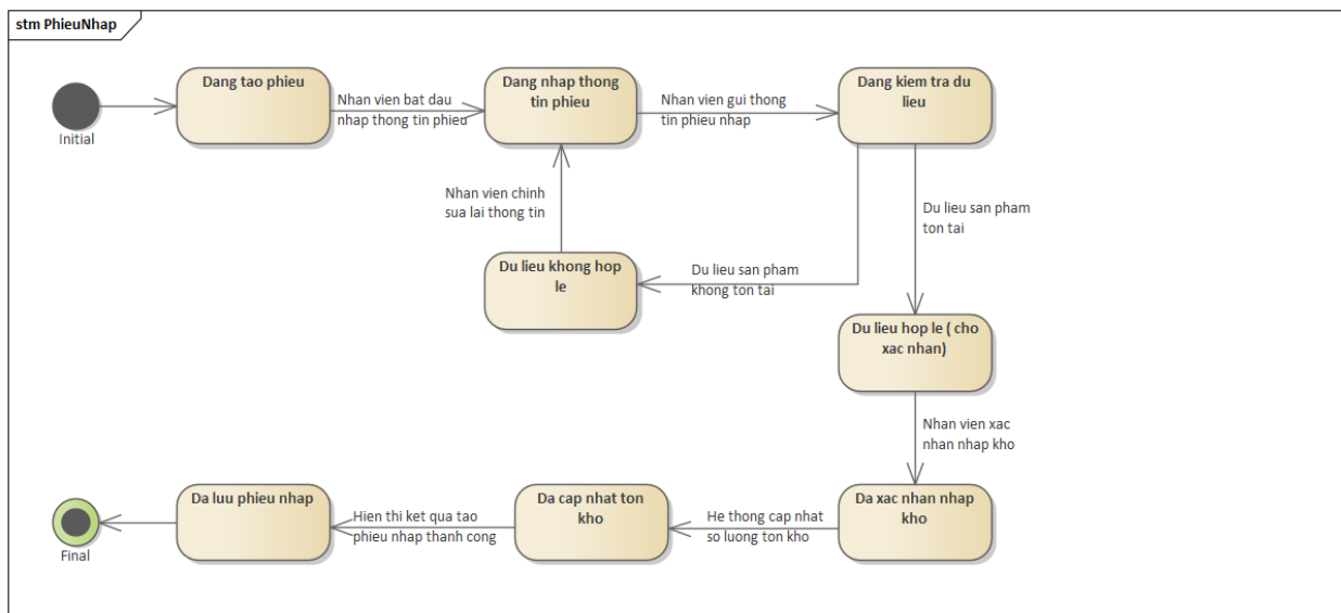
Hình 3. 22. Sơ đồ trạng thái Phiếu nhập
