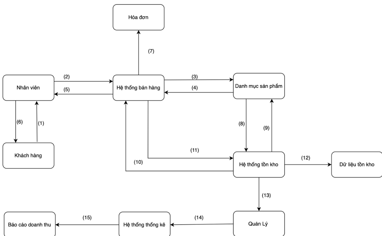
Hình 2. 1. Sơ đồ quy trình nghiệp vụ của cửa hàng bán lẻ
