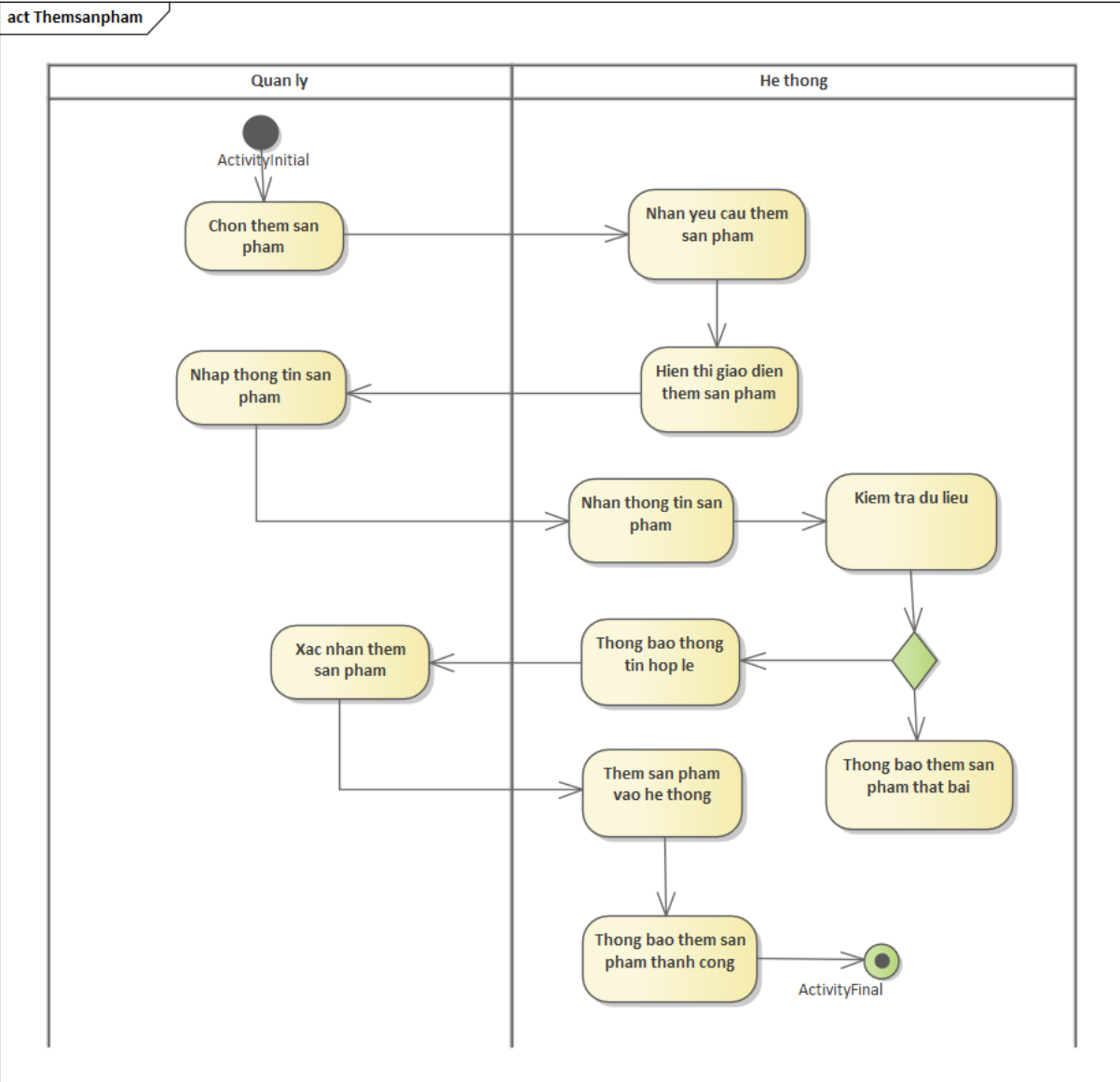
Hình 3. 2 Sơ đồ hoạt động Thêm sản phẩm
