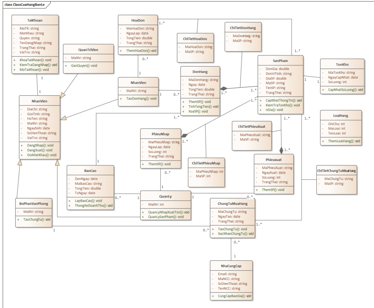
Hình 3. 20. Sơ đồ lớp
