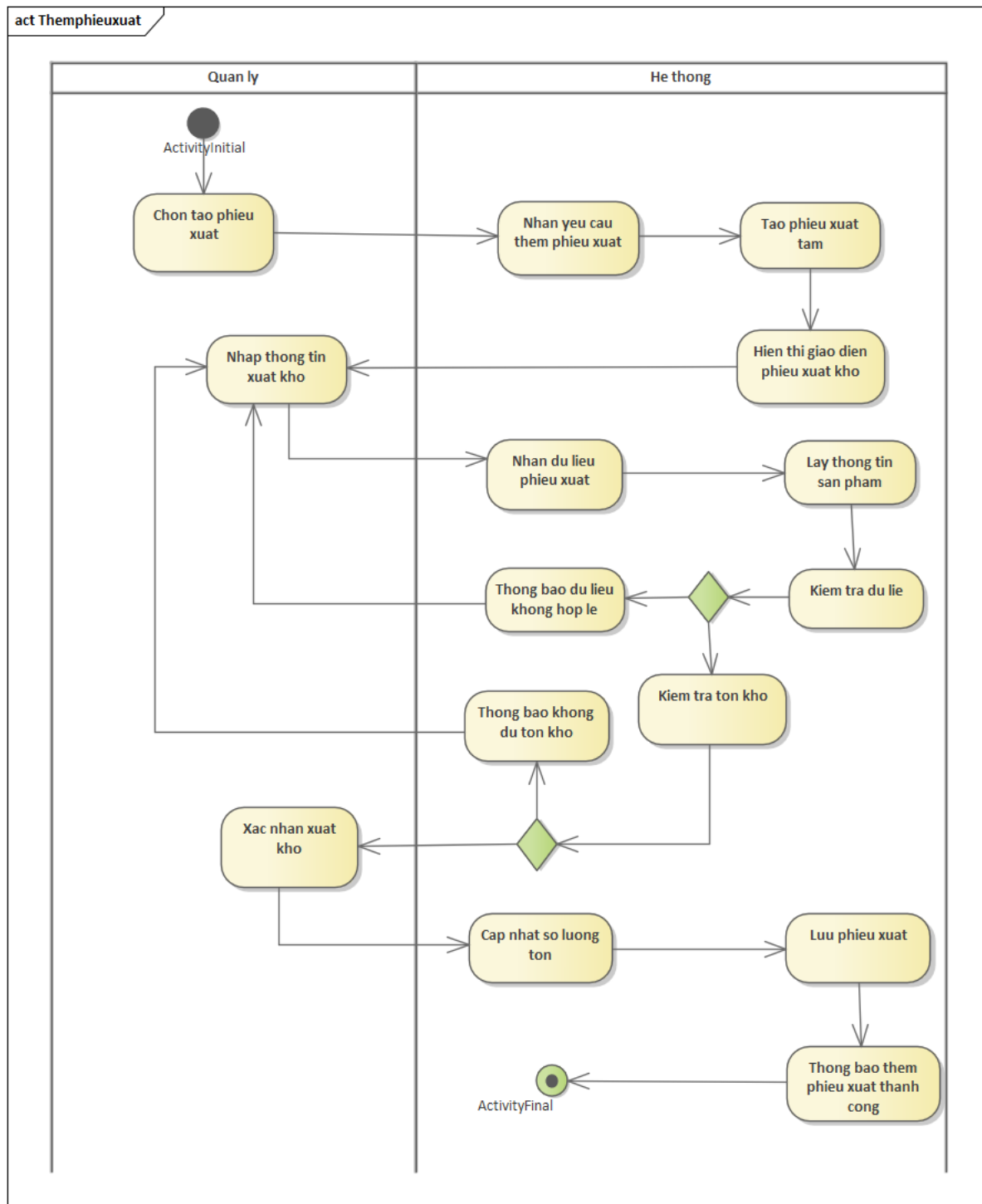
Hình 3. 3 Sơ đồ hoạt động Thêm phiếu xuất
