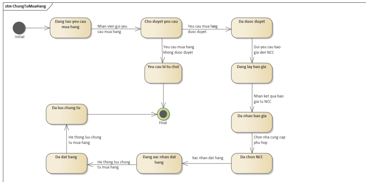
Hình 3. 24. Sơ đồ trạng thái Chứng từ mua hàng
