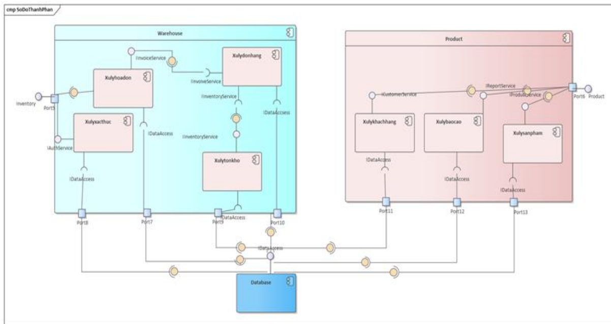
Hình 4. 19. Sơ đồ thành phần
