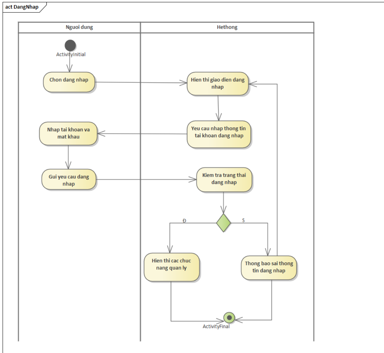
Hình 3. 1 Sơ đồ hoạt động Đăng nhập
