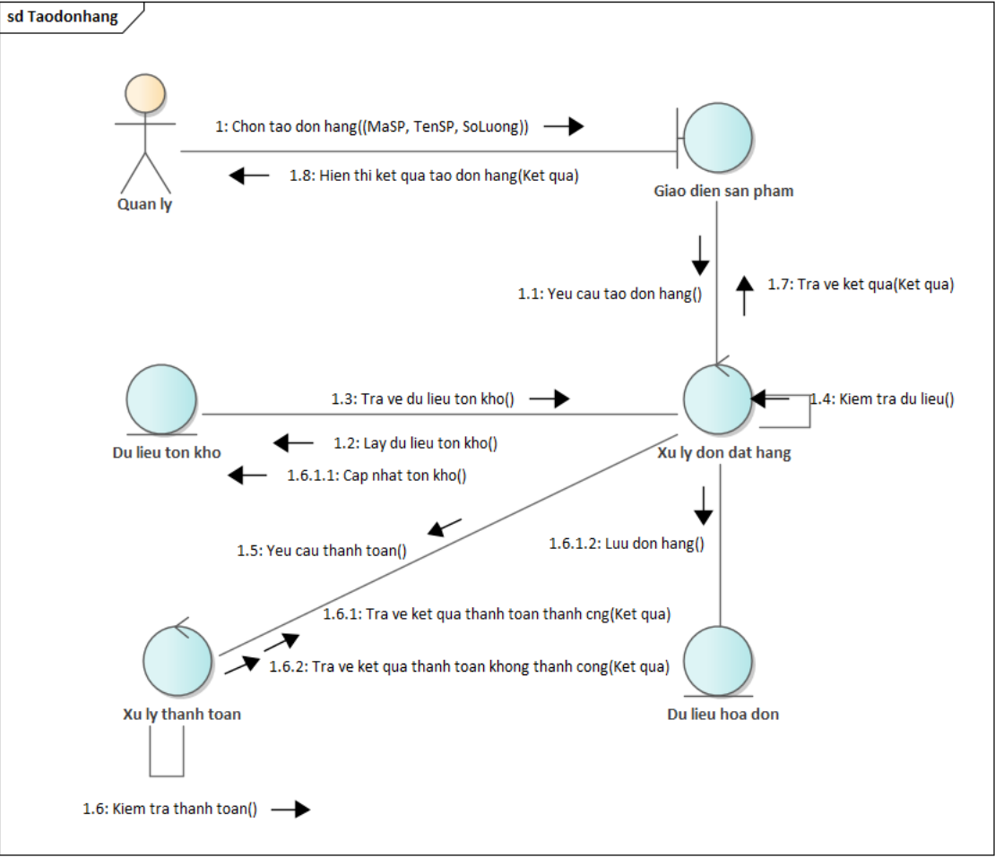
Hình 3. 16 Sơ đồ cộng tác tạo đơn hàng
