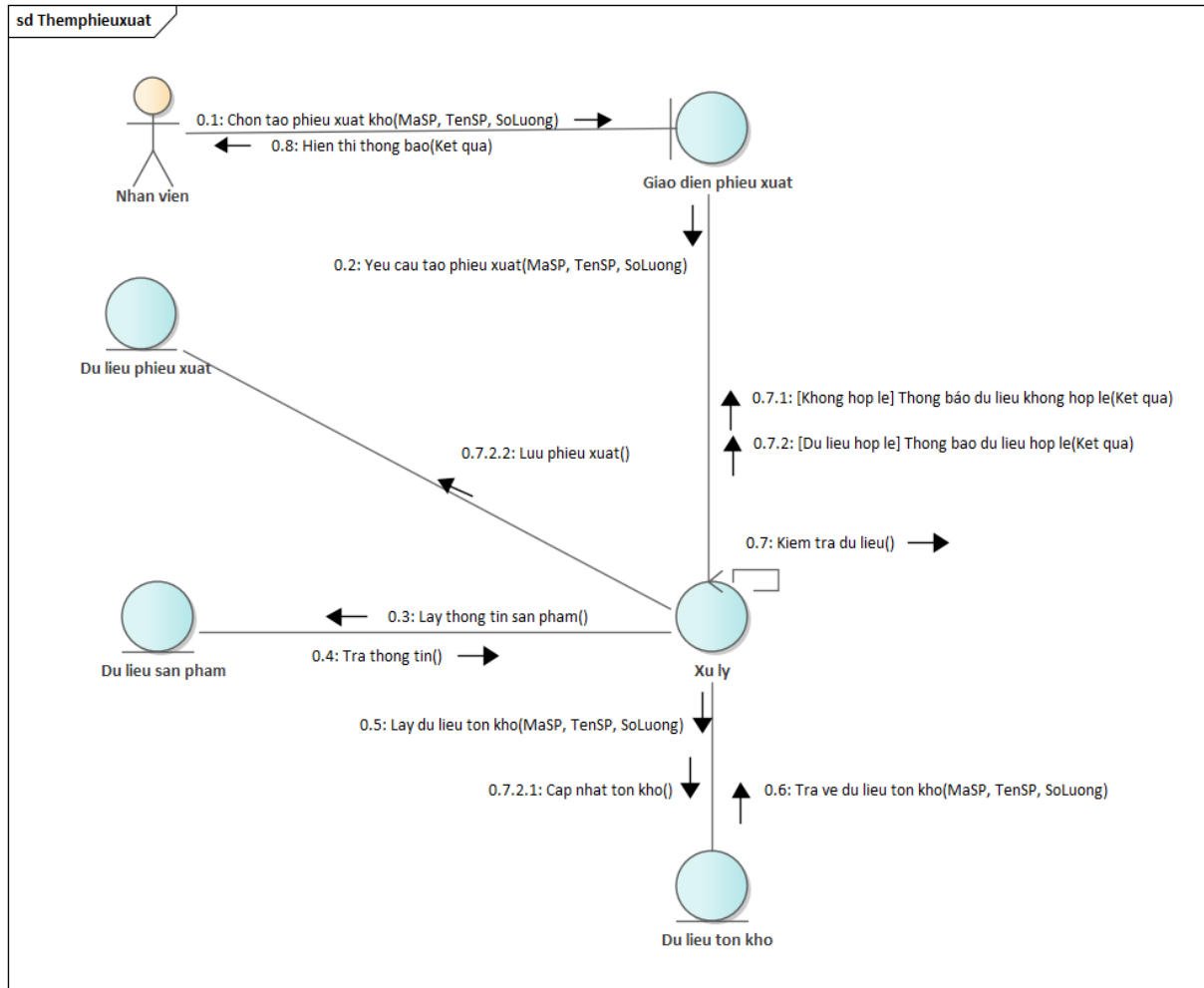
Hình 3. 15 Sơ đồ cộng tác Thêm phiếu xuất
