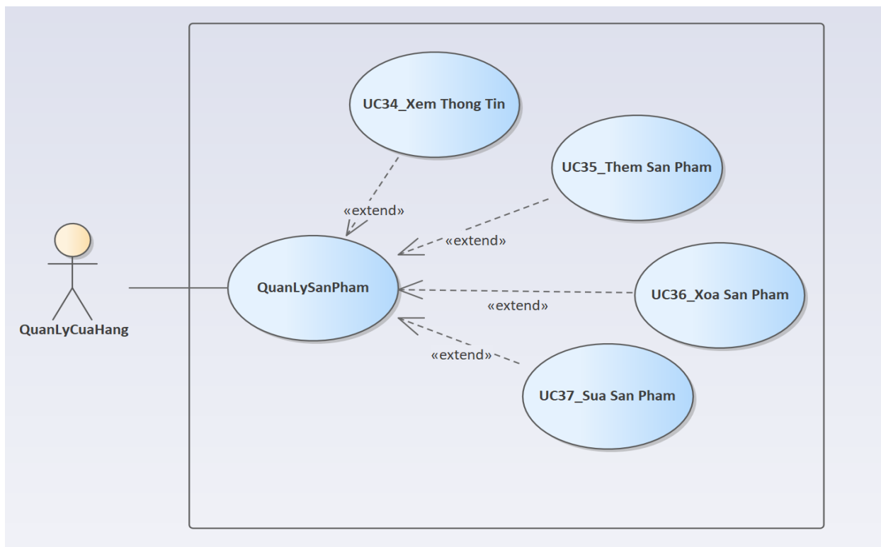
Hình 2. 8. Sơ đồ Use Case Quản lý sản phẩm
