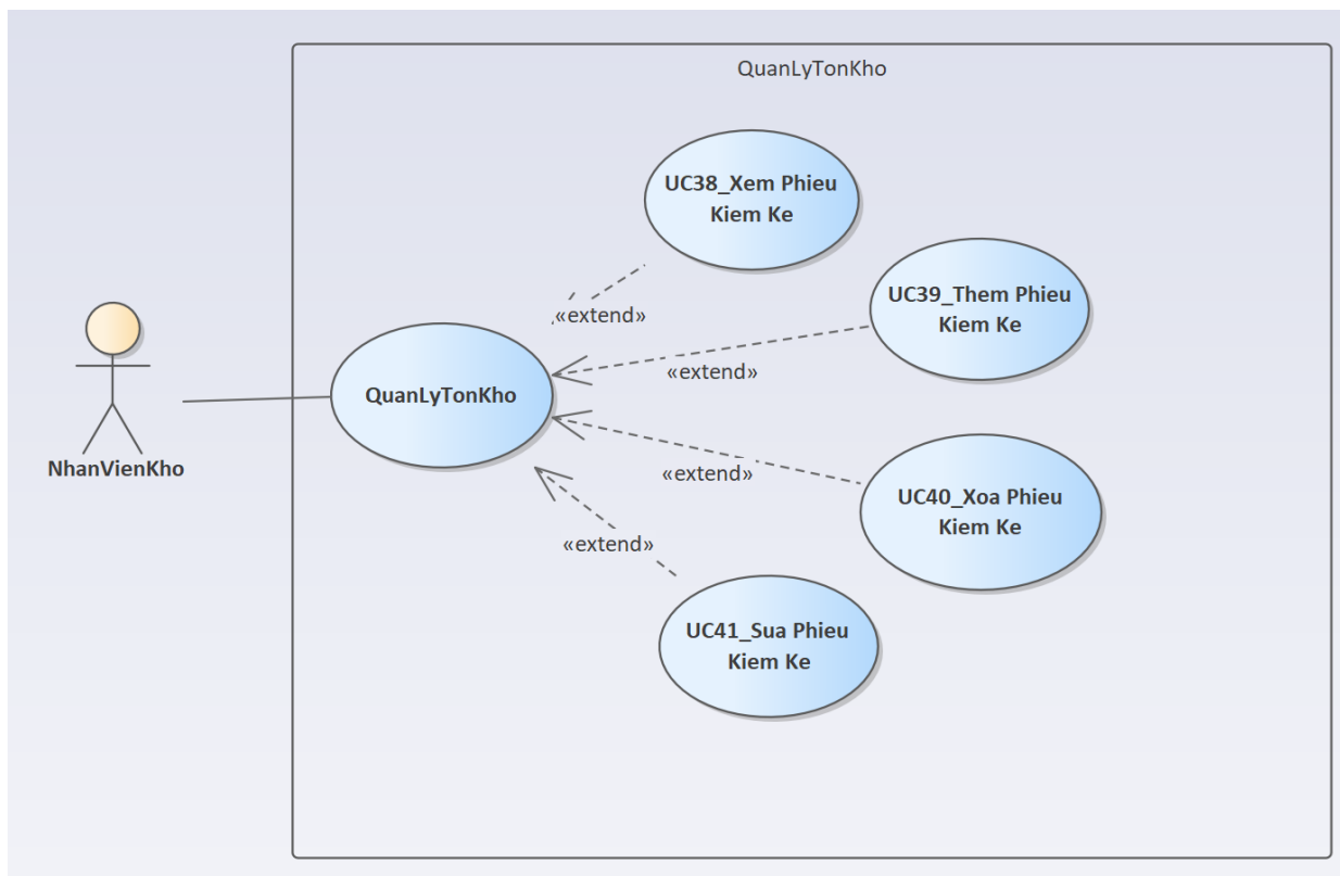
Hình 2. 7. Sơ đồ Use Case Quản lý tồn kho
