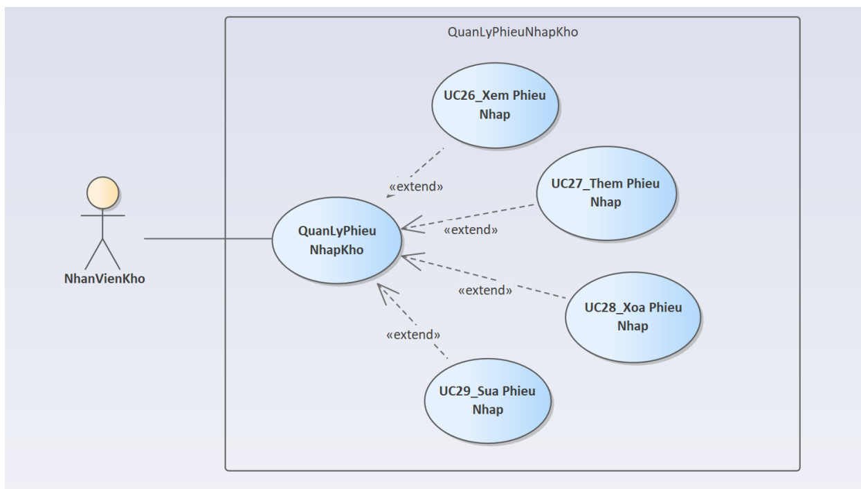
Hình 2. 10. Sơ đồ Use Case Quản lý phiếu nhập
