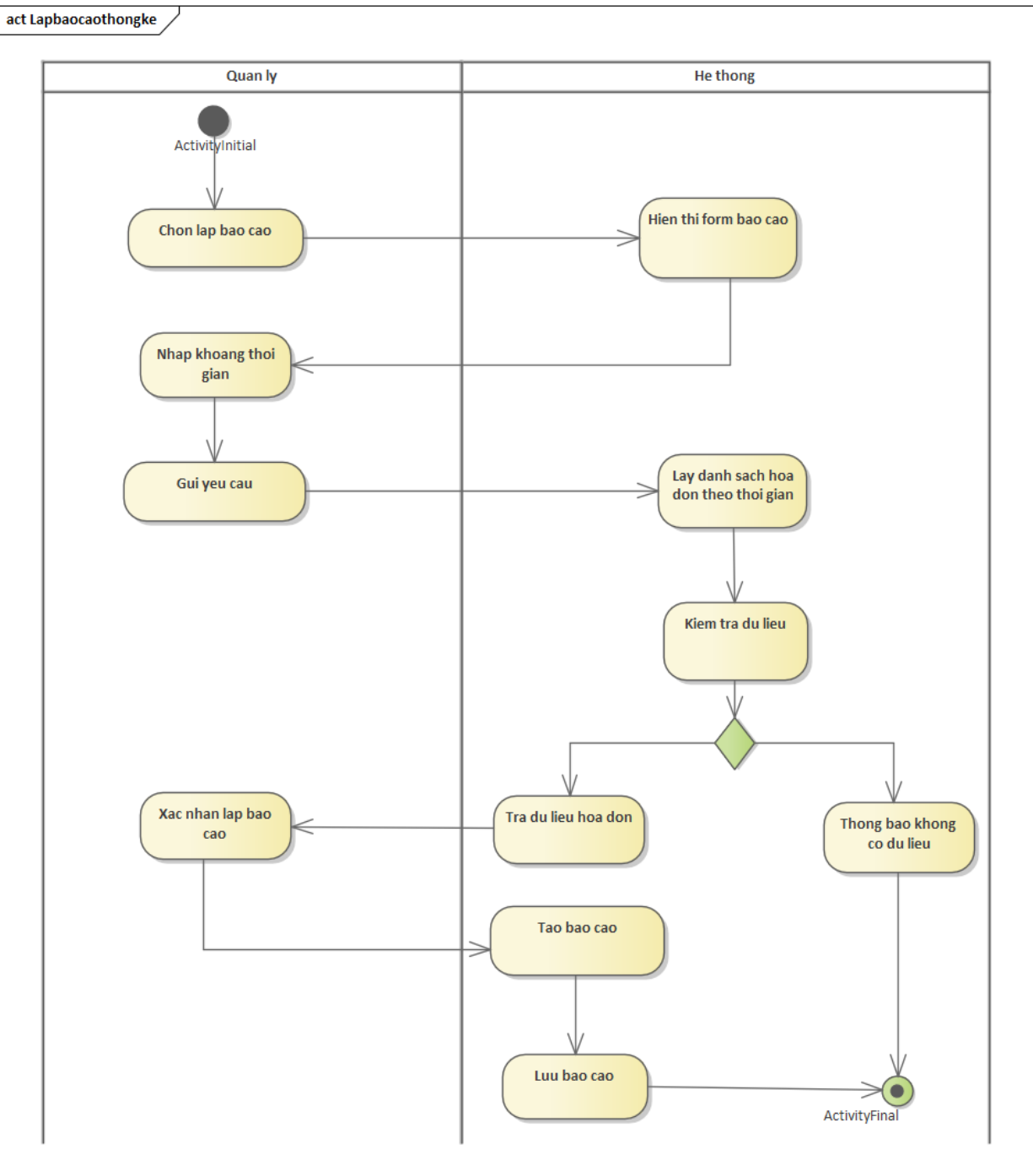
Hình 3. 6 Sơ đồ hoạt động Lập báo cáo thống kê
