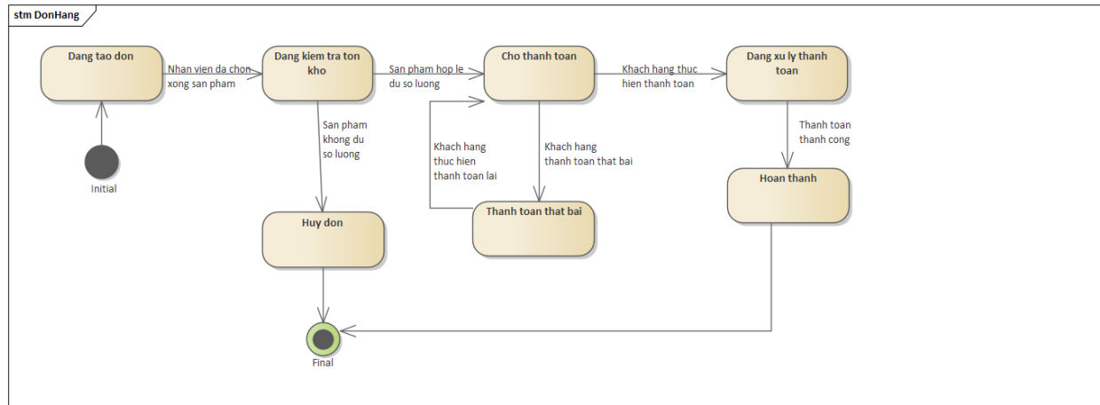
Hình 3. 23. Sơ đồ trạng thái Đơn hàng
