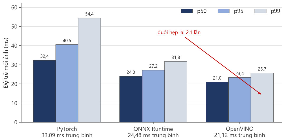
Hình 5.2. Độ trễ bộ phát hiện trên ba nền tảng suy luận CPU, tách theo phân vị. Khoảng cách giữa ba nền tảng giãn ra khi đi từ p50 sang p99 — đó là dấu hiệu OpenVINO không chỉ nhanh hơn mà còn ổn định hơn .
