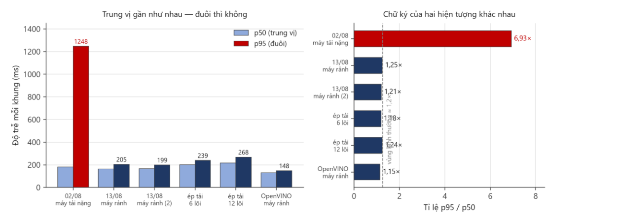
Hình 5.3. Sáu lần đo NFR-P2. Bên trái: trung vị của lượt đo cũ nằm ngang với các lần đo trên máy rãnh, nhưng đuôi p95 cao gấp sáu lần. Bên phải: cùng dữ liệu, biểu diễn bằng tỉ lệ p95/p50 — ép tải tới 12 lõi cũng chỉ đẩy tỉ lệ này lên 1,24× trong khi lượt đo cũ là 6,93× . Tải cạnh tranh nâng cả phân bố đều tay; thứ xảy ra ở lượt đo cũ thì không.
