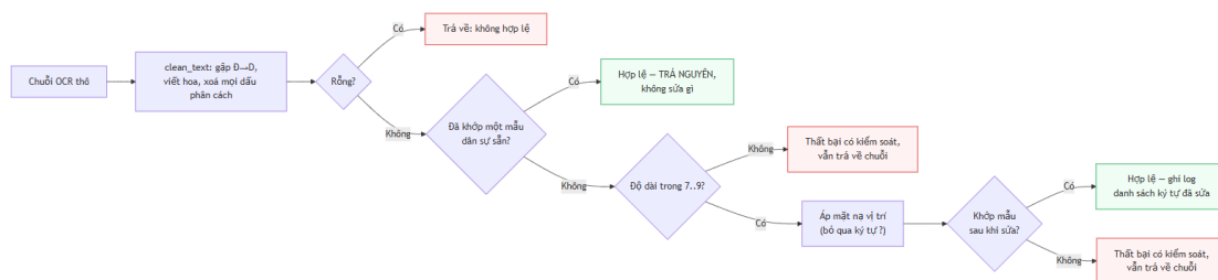
Hình 3.4. Thuật toán chuẩn hoá chuỗi biển số theo bộ luật ràng buộc vị trí
