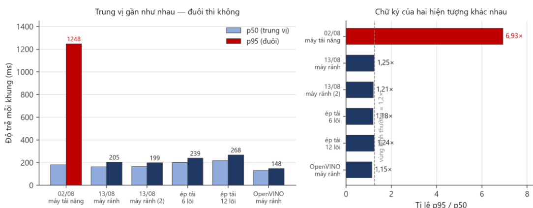
Hình 5.3. Sáu lần đo NFR-P2. Trung vị của lượt đo cũ nằm ngang với các lần đo trên máy rảnh, nhưng đuôi p95 cao gấp sáu lần; ép tải tới 12 lõi cũng chỉ đẩy tỉ lệ p95/p50 lên 1,24× trong khi lượt đo cũ là 6,93× .
