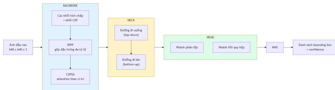
Hình 2.1. Kiến trúc tổng quát backbone – neck – head của YOLO11 (theo [14], [10])
