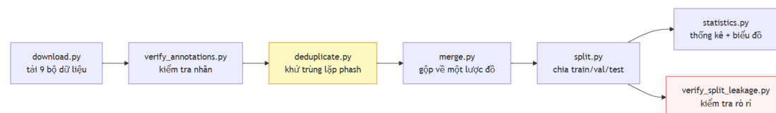
Hình 3.2. Đường ống sáu bước xây dựng bộ dữ liệu
