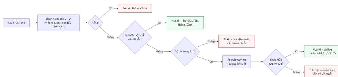
Hình 4.6. Thuật toán chuẩn hoá chuỗi biển số theo bộ luật ràng buộc vị trí
