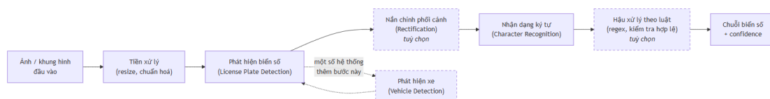
Hình 2.1. Sơ đồ pipeline ALPR điển hình (tổng hợp từ [2], [3], [20], [22], [23])
