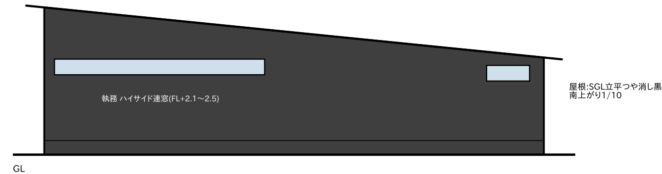
東立面図(生垣・水路側) 1/150
