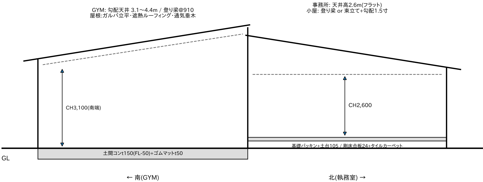
A-A断面図(南北) 1/60 ※雨仕舞い: GYM高壁と事務所低軒の取り合いは雨押え板金・両屋根とも接合部から離れる方向に排水
