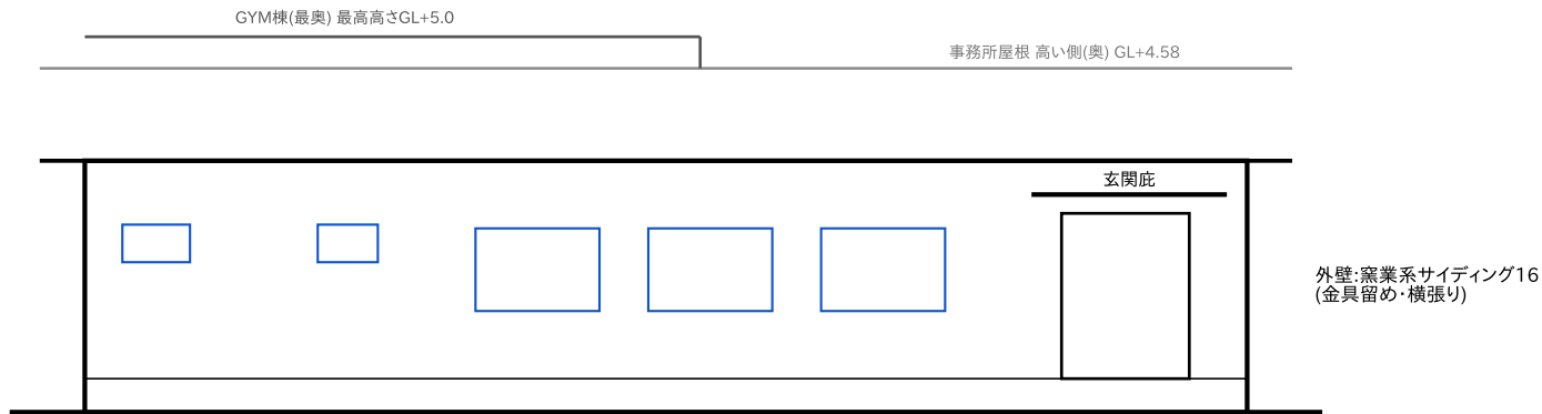
北立面図(道路側) 1/150
