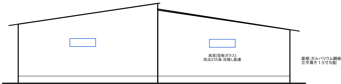
(GYM東面は事務所面より7.3m奥) 東立面図(水路側) 1/150
