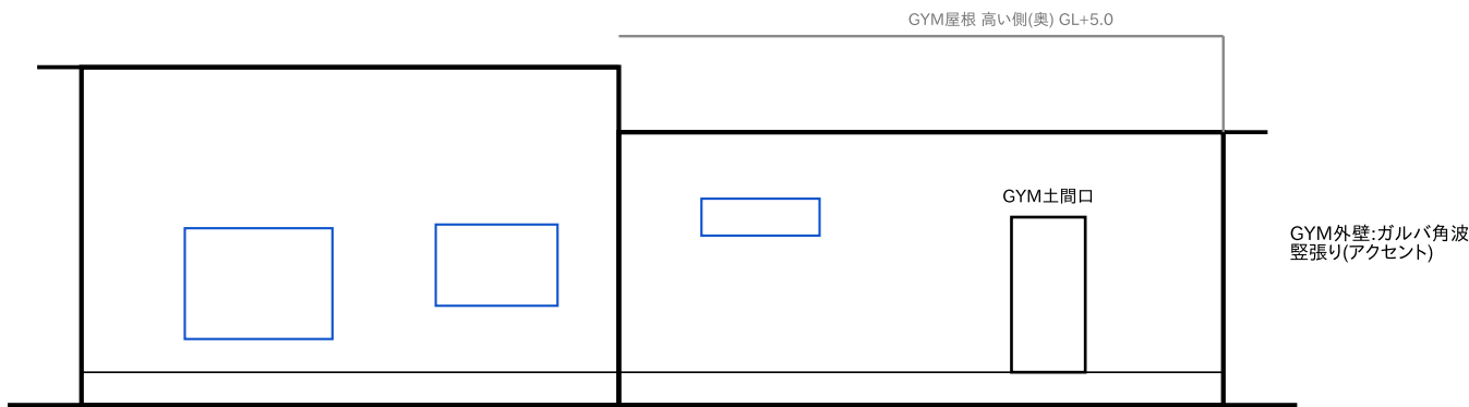
南立面図 1/150
