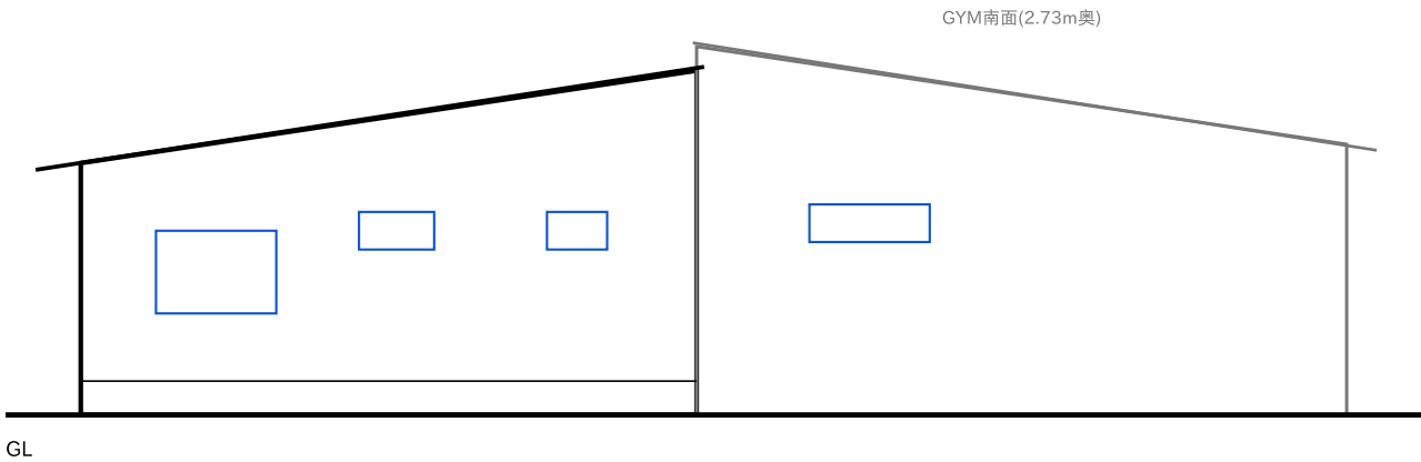
南立面図 1/150
