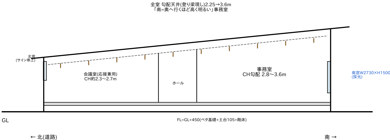
A-A断面図(南北・x=2.3 会議室～ホール～事務室) 1/60
