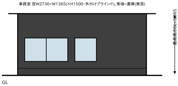
南立面図(採光面) 1/150
