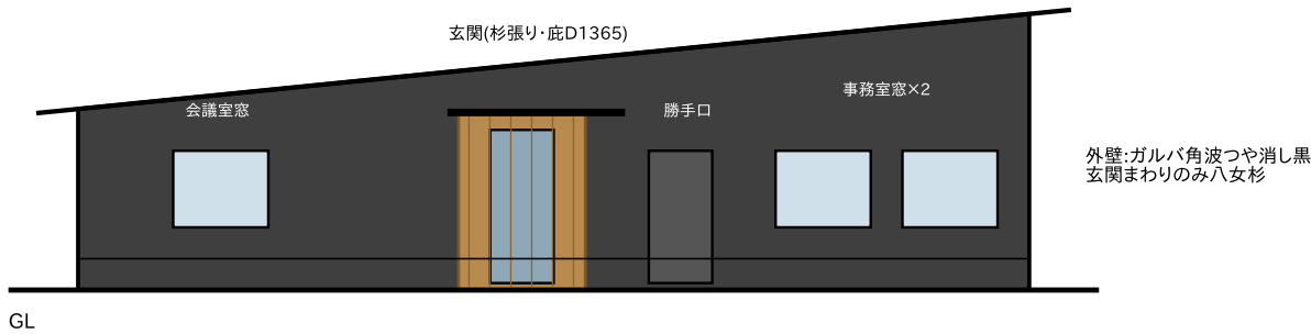
西立面図(ヤード・駐車場側=入口の顔) 1/150
