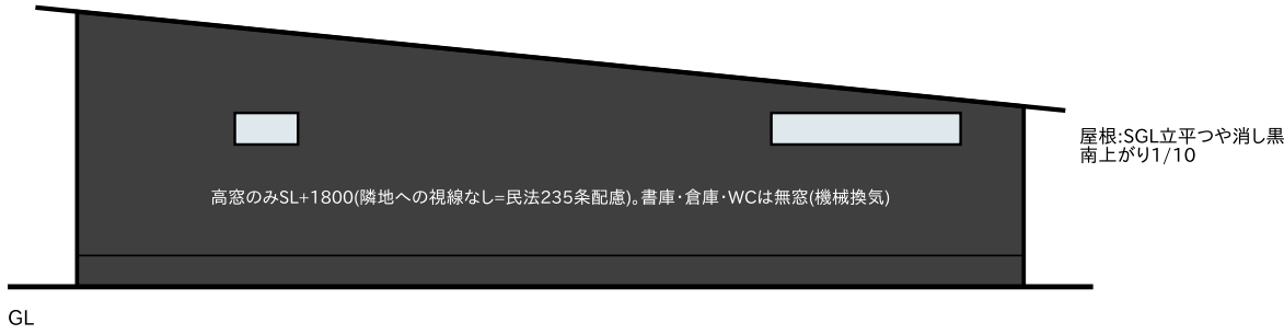
東立面図(生垣・水路側) 1/150
