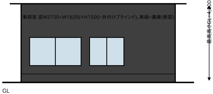
南立面図(採光面) 1/150
