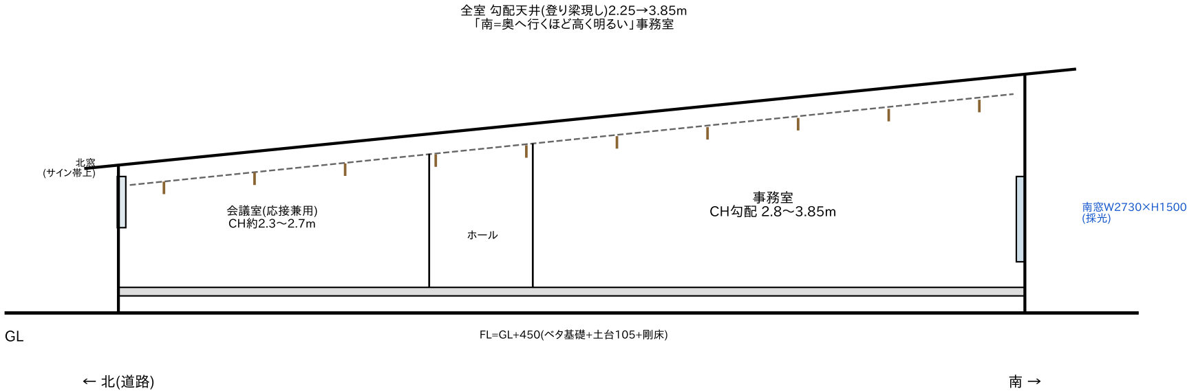
A-A断面図(南北・x=2.3 会議室～ホール～事務室) 1/60
