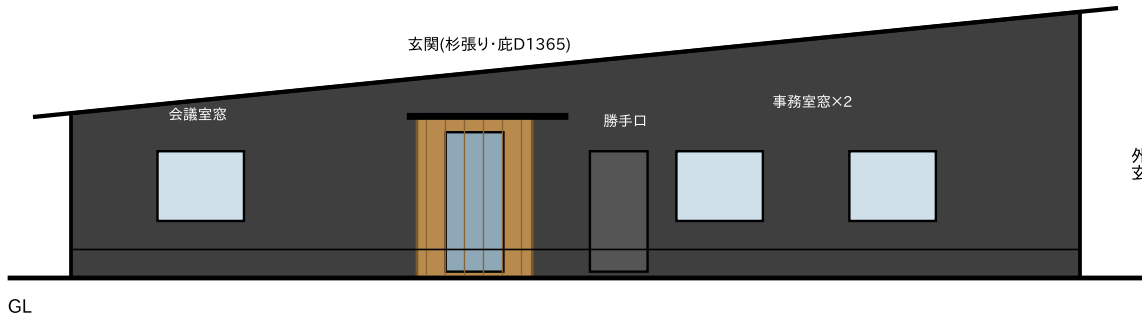
西立面図(ヤード・駐車場側=入口の顔) 1/150
