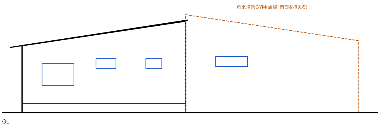
南立面図 1/150
