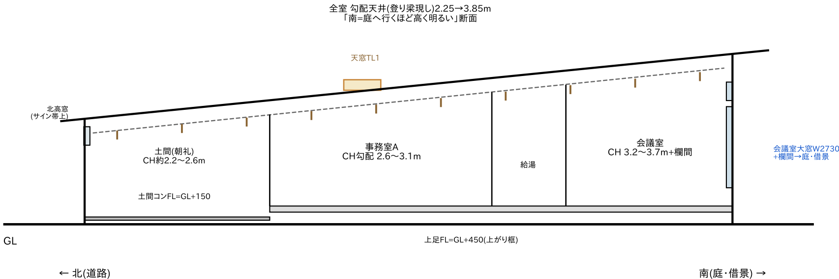
A-A断面図(南北・x=3.0 土間~事務A~給湯~会議室) 1/60
