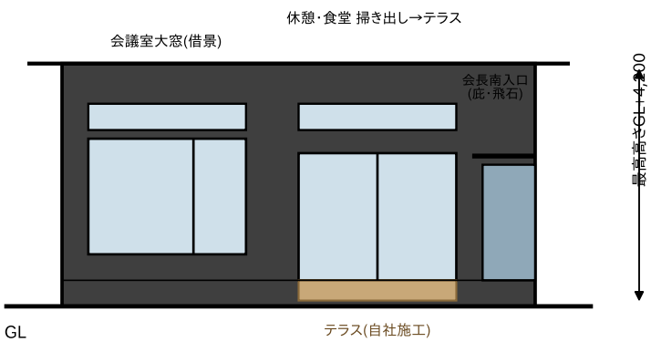
南立面図(庭・借景側) 1/150
