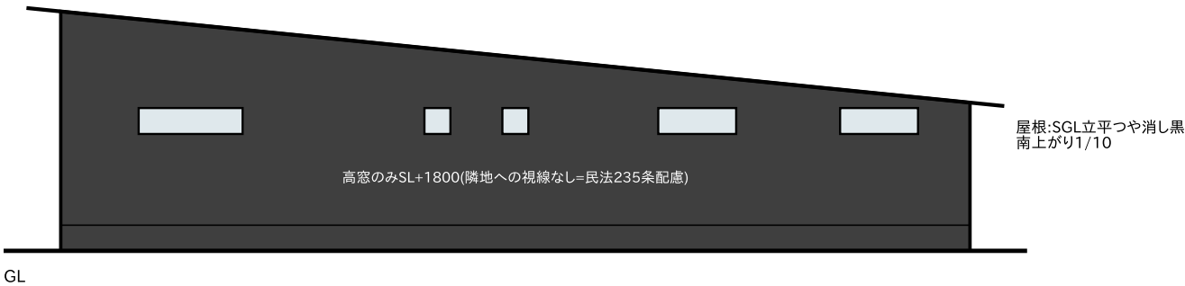
東立面図(生垣・水路側) 1/150
