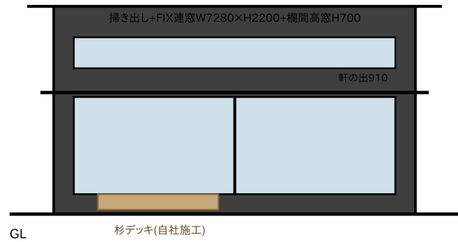
南立面図(庭・借景側) 1/150
