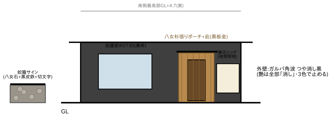
北立面図(道路の顔) 1/150
