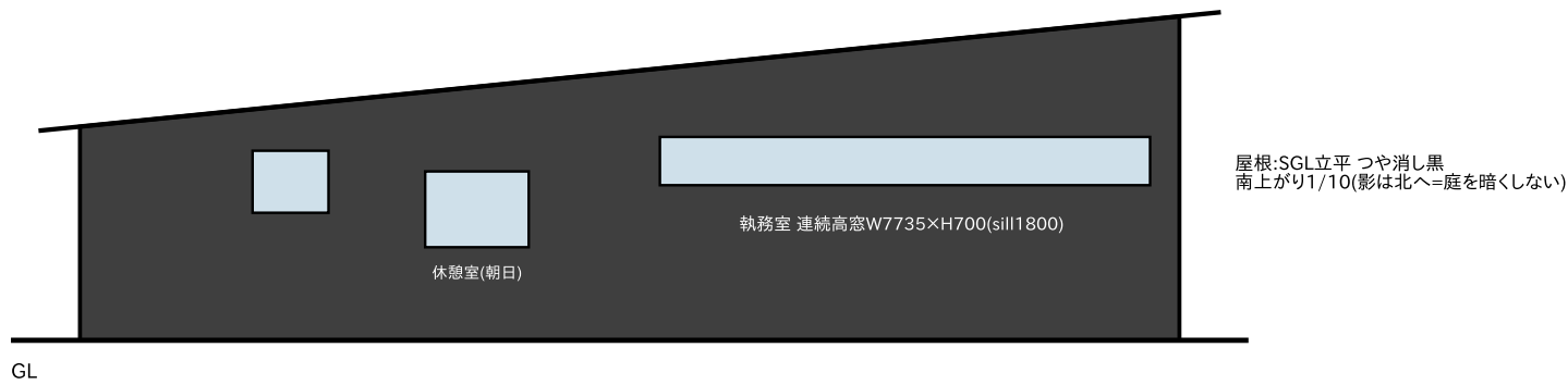
東立面図(生垣・水路側) 1/150
