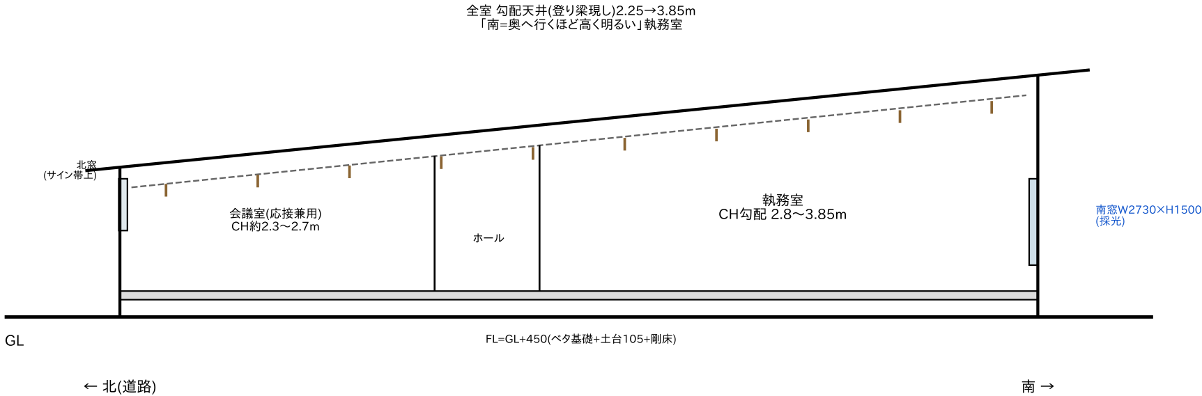
A-A断面図(南北・x=2.7 会議室～ホール～執務室) 1/60
