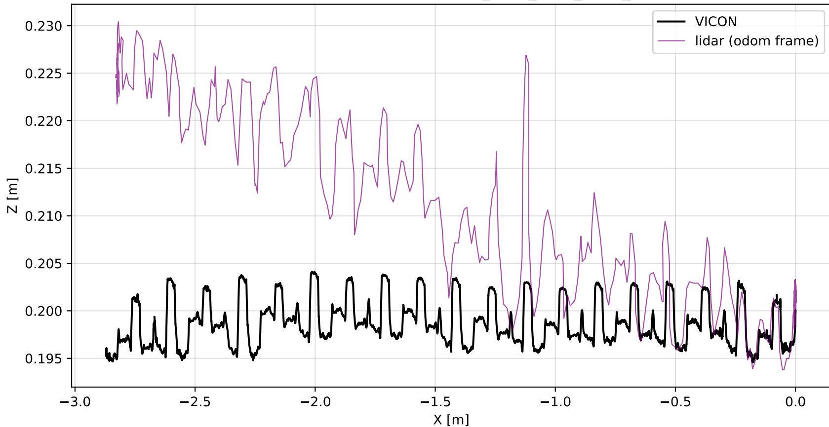
LiDAR XZ Trajectory — FLAT_WLW_NEW_REAL_2
