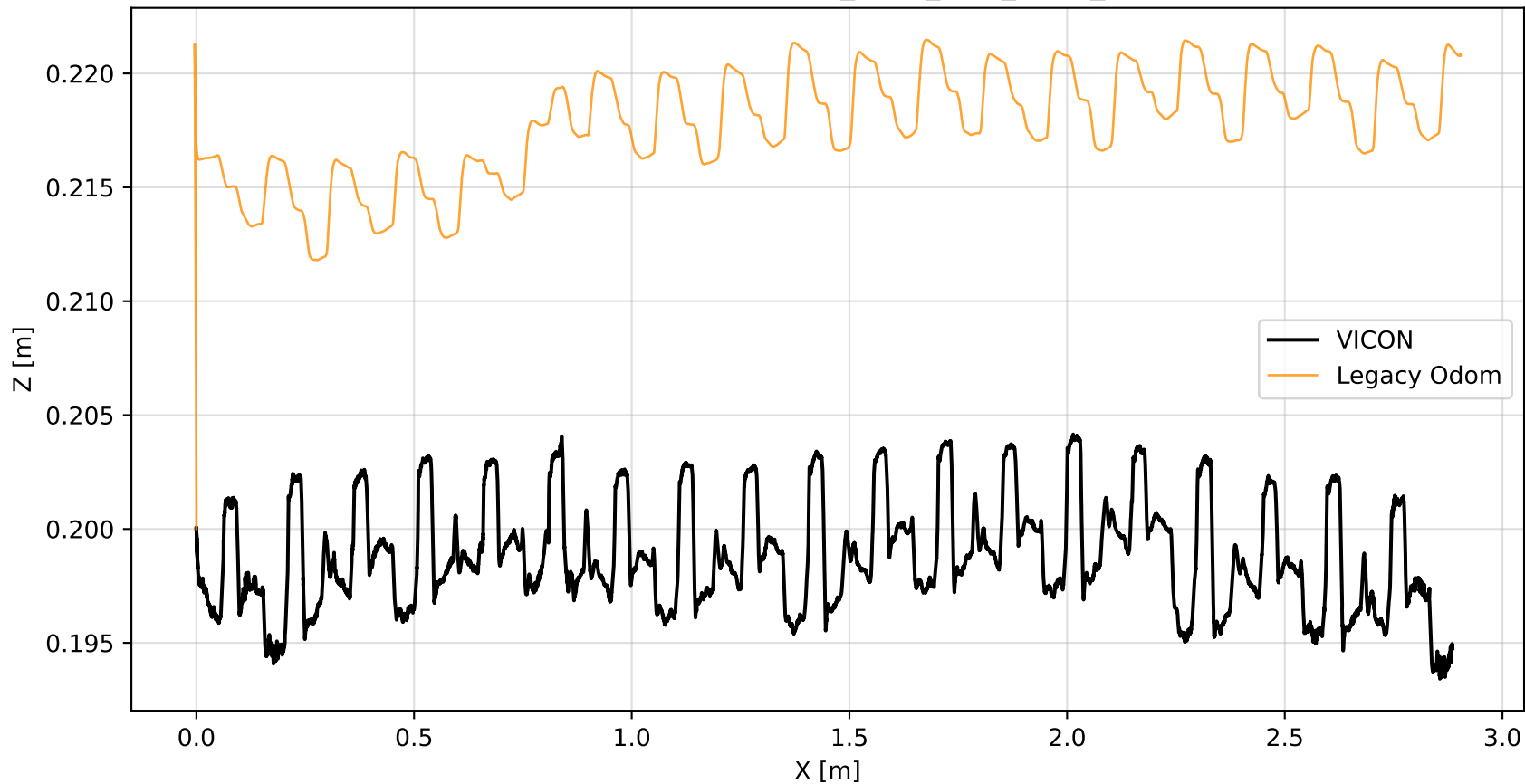
XZ Trajectory — FLAT_WLW_OLD_REAL_5
