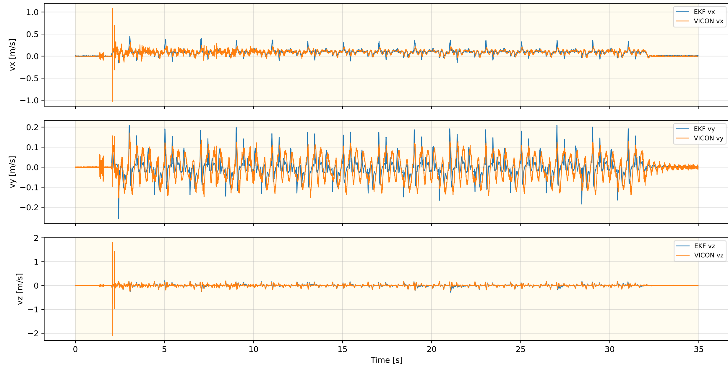
Inner EKF Velocity — FLAT_Walk_NEW_REAL_4
