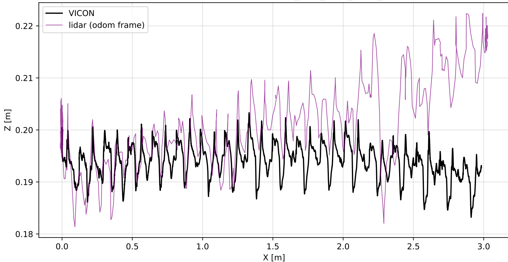
LiDAR XZ Trajectory — FLAT_MPC_NEW_REAL_3
