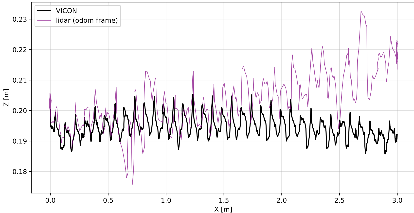
LiDAR XZ Trajectory — FLAT_MPC_NEW_REAL_5
